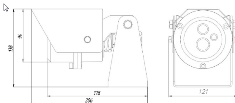
Рисунок 4.1 – Габаритные размеры термокожуха
