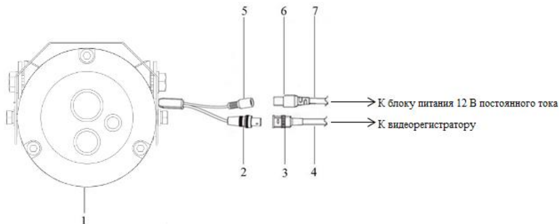
Рисунок 4.3 - Схема подключения термокожуха с сетевым видеомодулем
