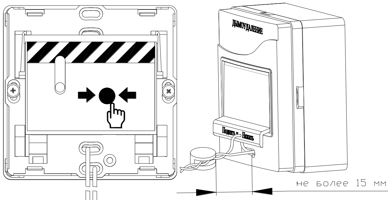
Рисунок 2.2.3.2 Пломбировка УДП
