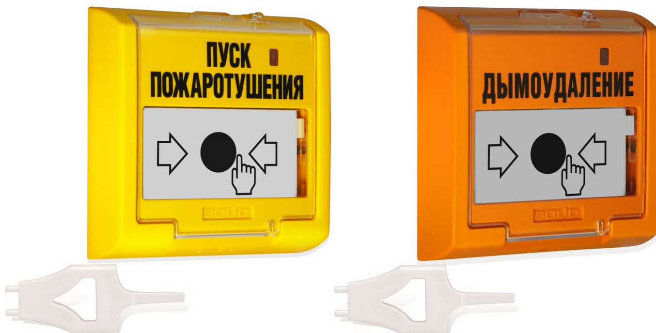
Рисунок 2.2.2.1 Внешние виды «УДП 513-3АМ» и «УДП 513-3АМ исп.02»
