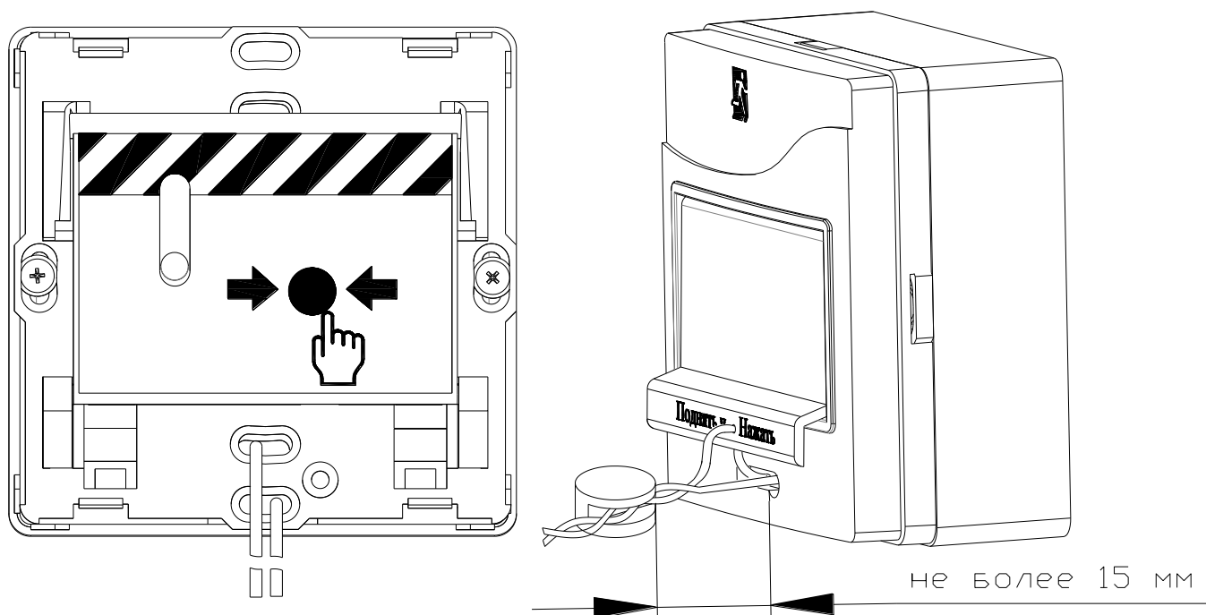
Рисунок 2.2.3.2 Пломбировка УДП
