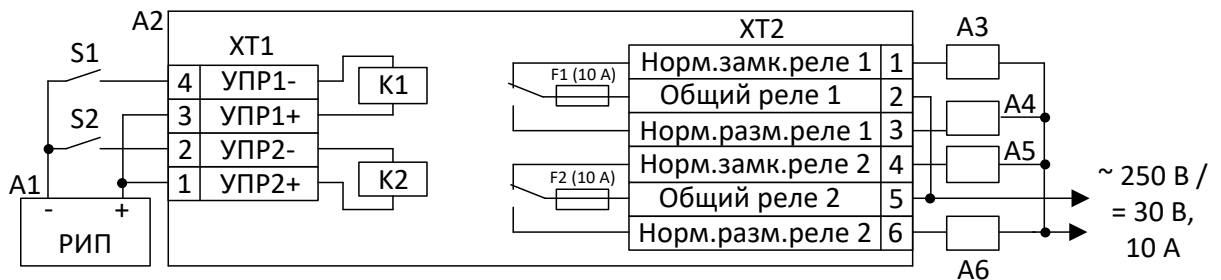
Рис.2 Схема подключения УК-ВК исп.12, исп.13, исп.14, исп.15
