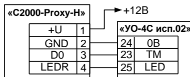
Рисунок 7. Схемы подключения считывателей
