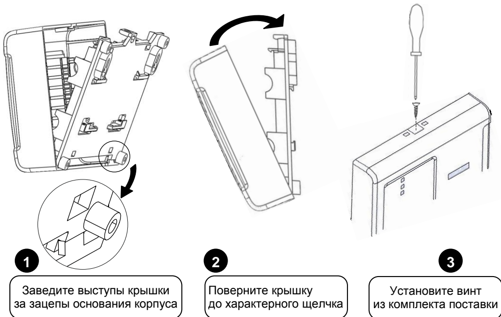
Рисунок 4. Установка крышки прибора
