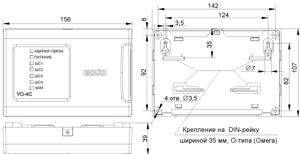
Рисунок 1. Габаритные и установочные размеры «YO-4C исп.02»
