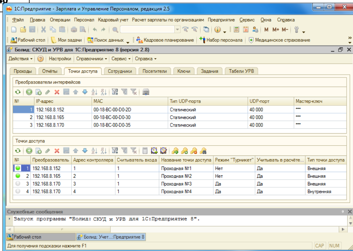
Рисунок 3.19. Страница «Точки доступа».
