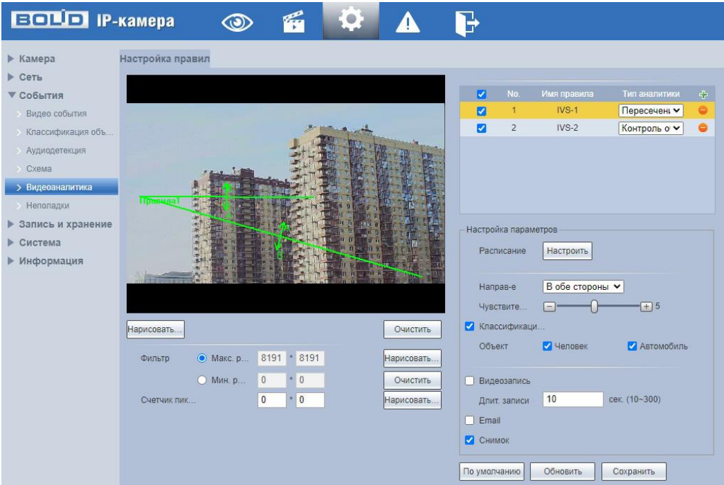
Рисунок 7.79 – Создание правила видеоаналитики «Пересечение линии»
