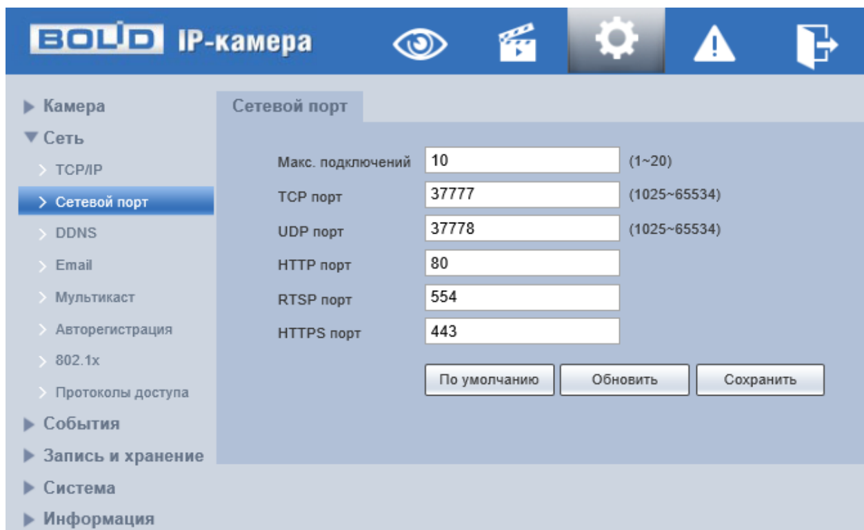
Рисунок 7.54 – Подпункт меню «Сетевой порт»
