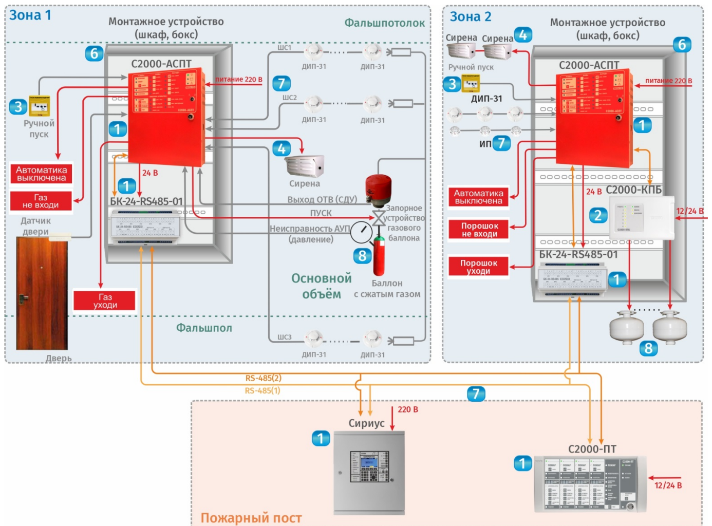
Рис. 3. Структурная схема АУП с блоками С2000-АСПТ
