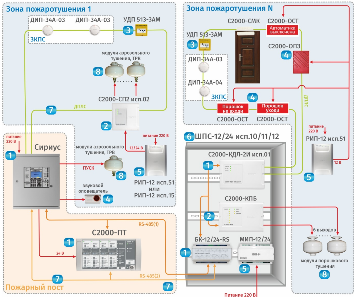
Рис. 2. Структурная схема АУПП, АУАП, АУП-ТРВ
