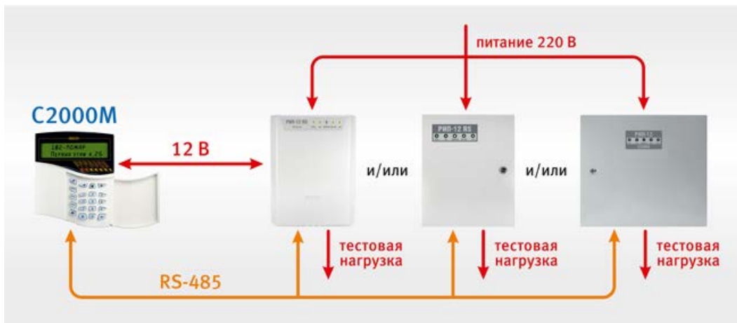
Рис. 195.Схема установки для испытаний
