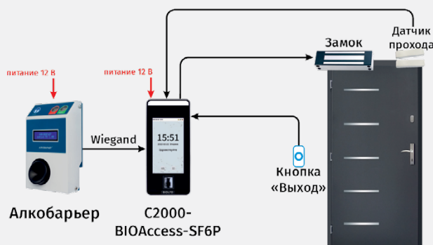
Рисунок 67. Подключение алкотестеров к биометрическим контроллерам
