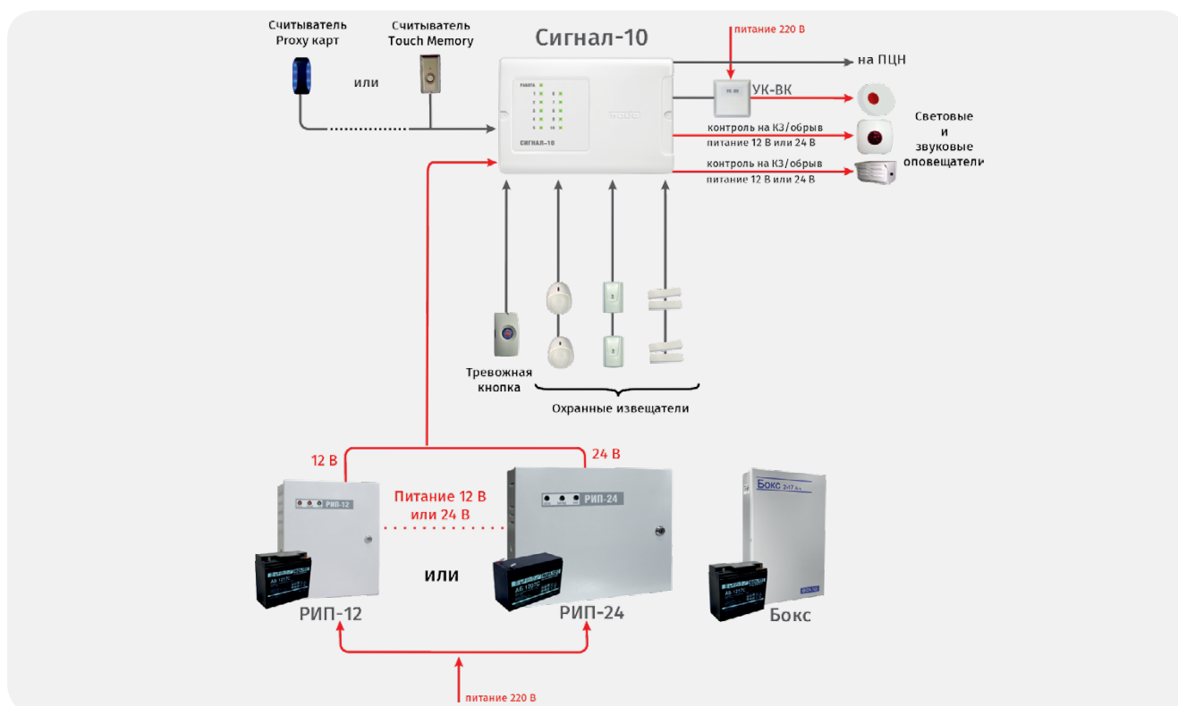
Рисунок 44. Автономное использование прибора «Сигнал-10»
