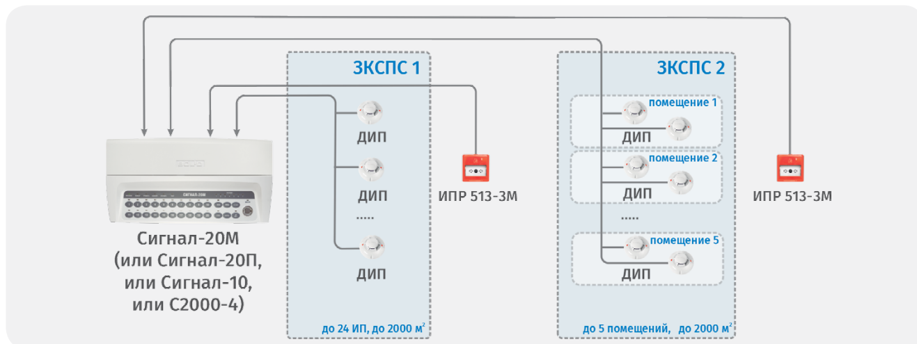
Рисунок 2. Организация линий и ЗКСПС в неадресных СПС
