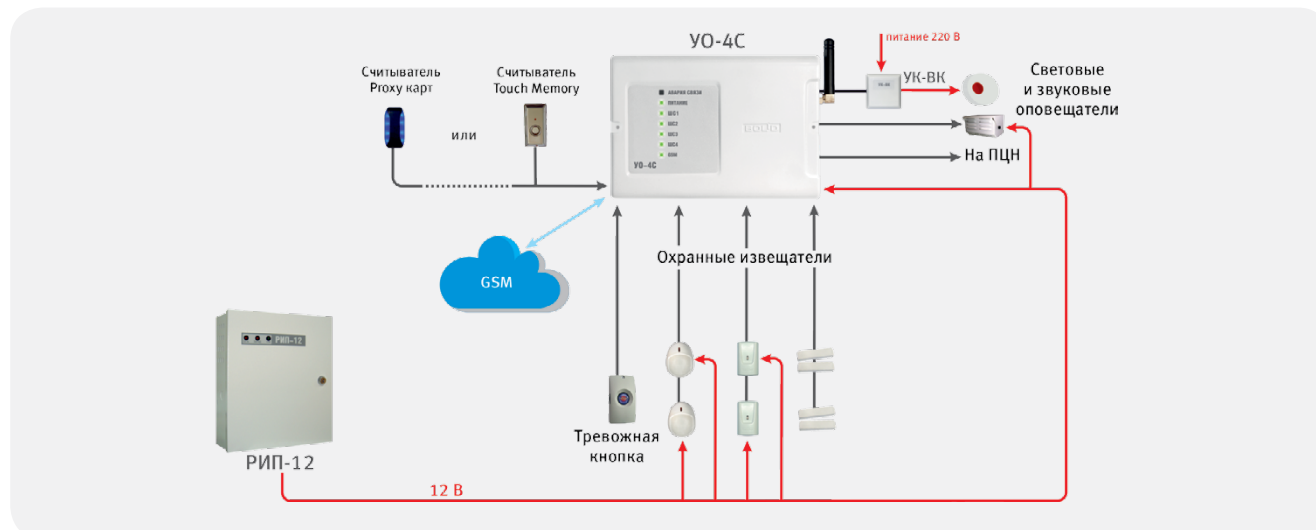
Рисунок 46. Автономное использование «YO-4C»
