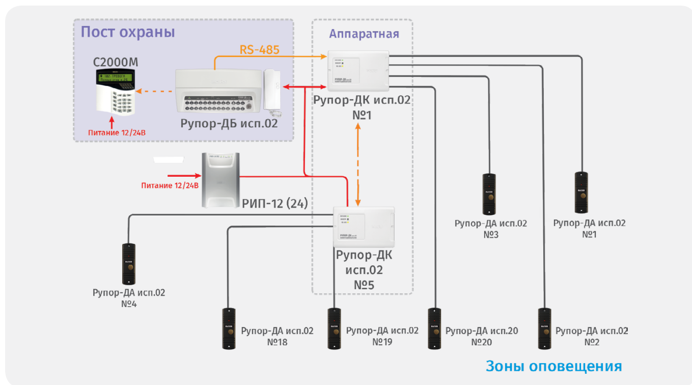
Рисунок 57. Система диспетчерской связи
