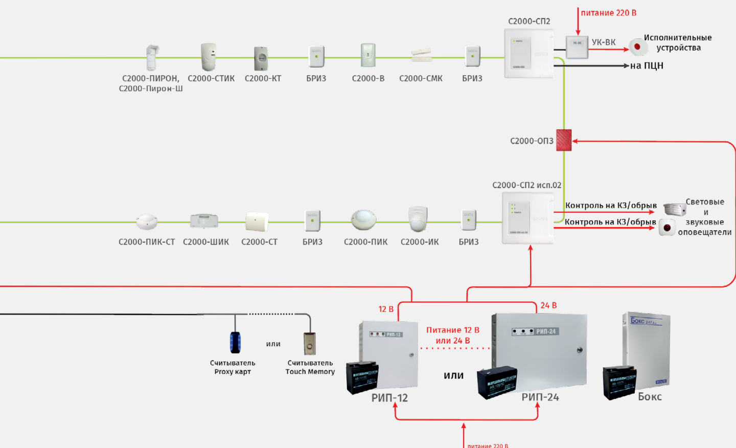
Рисунок 49. Адресная система охранной сигнализации
