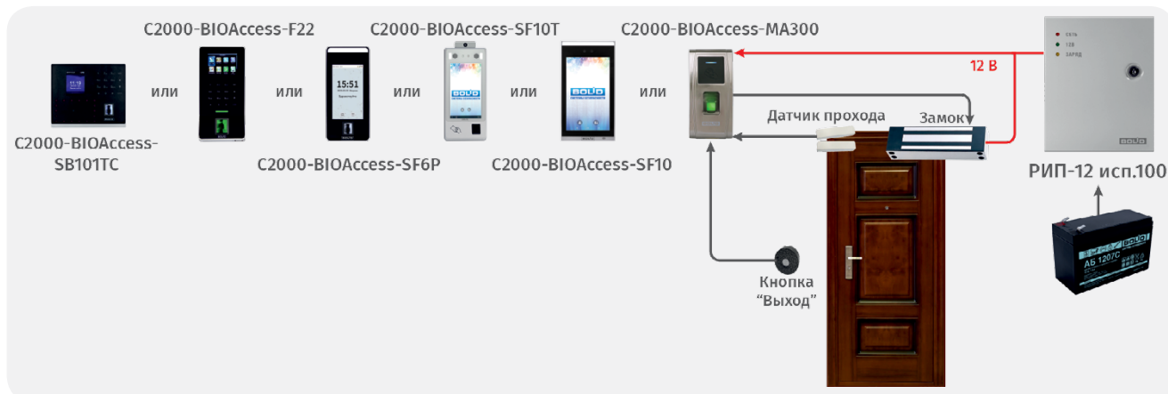
Рисунок 66. Биометрическая СКУД
