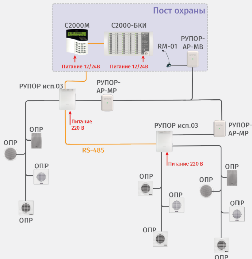
Рисунок 56. Система оповещения для малых и средних объектов
