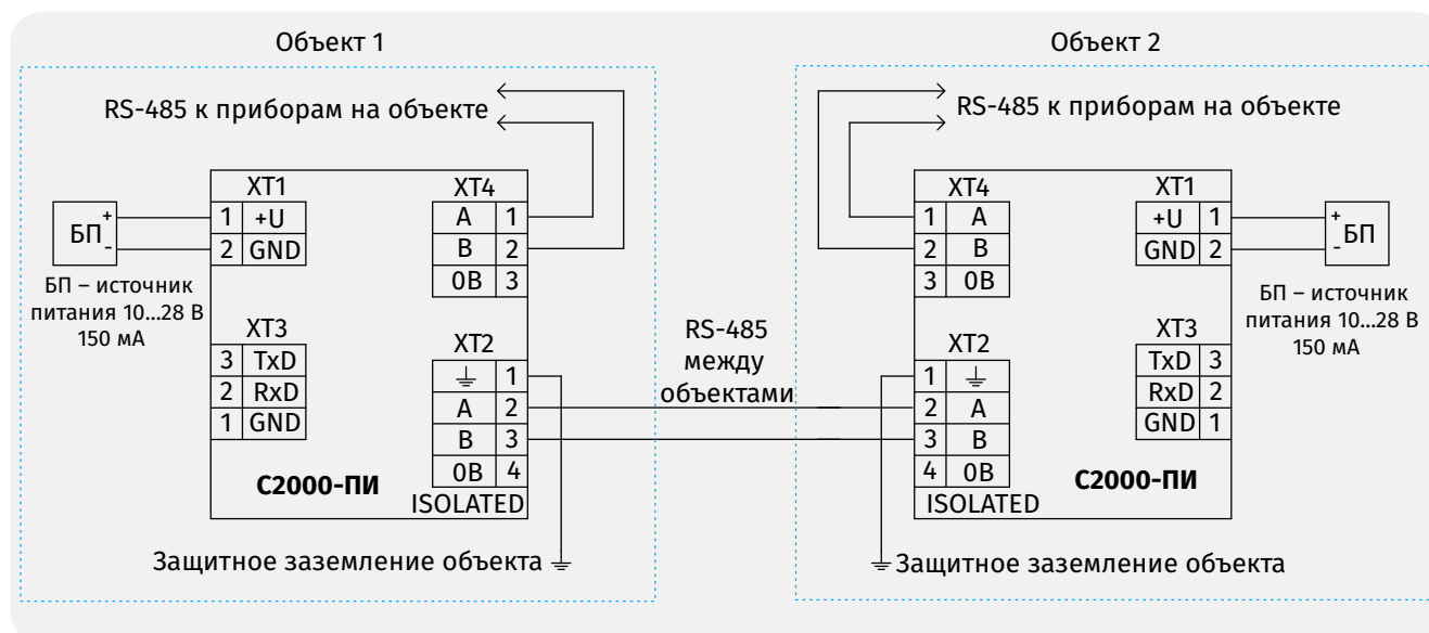
Рисунок 34. Схема подключения с защитой интерфейса RS-485 от перенапряжений
