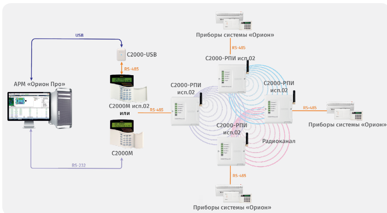
Рисунок 117. Структурная схема использования «С2000-РПИ исп.02» с «С2000М»/ «С2000М исп.02»
