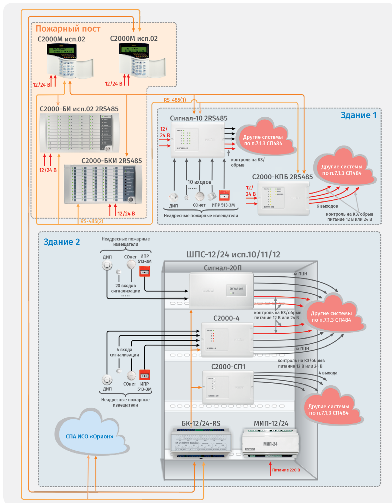
Рисунок 7. Распределенная неадресная СПС на базе пульты C2000M исп.02
