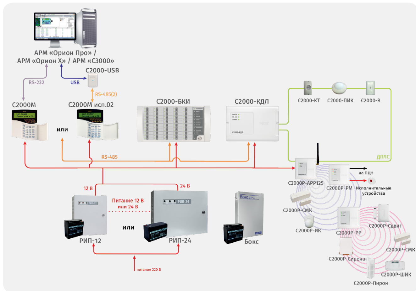
Рисунок 50. Адресная радиоканальная система на основе «C2000P-APP125»
