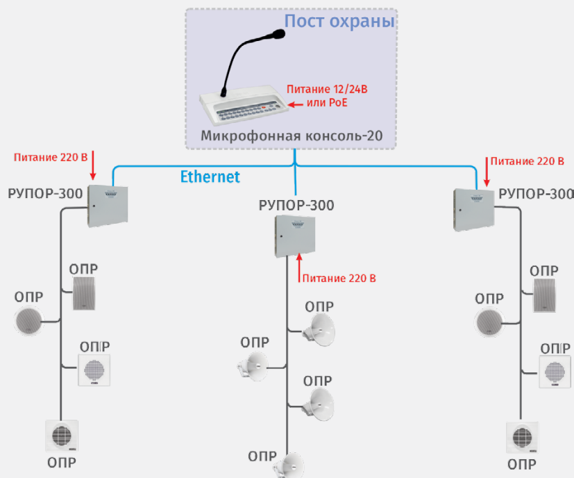
Рисунок 55. Система оповещения для больших объектов
