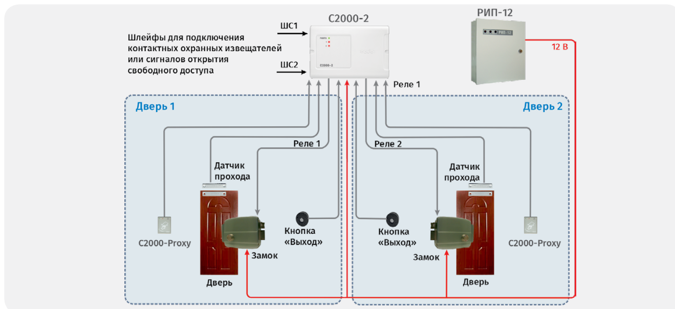
Рисунок 58. Режим работы «Две двери на вход»
