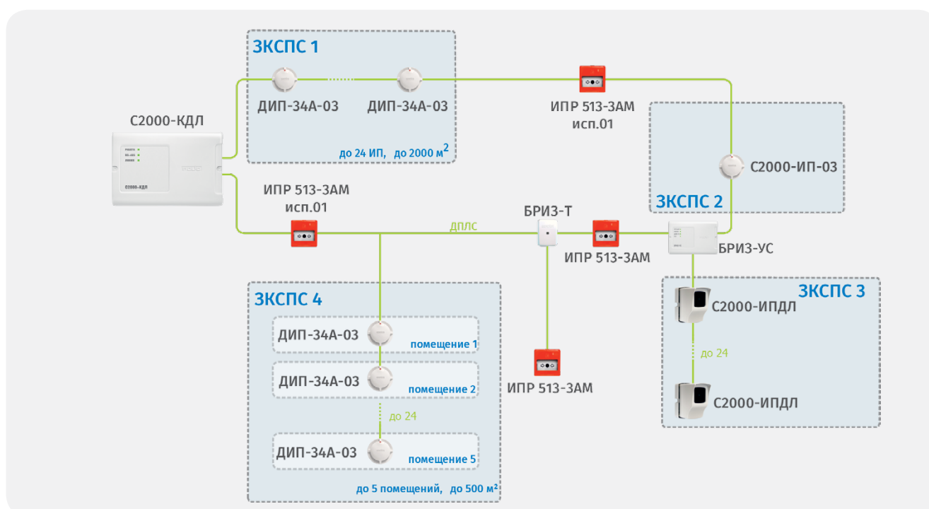
Рисунок 4. Организация ДПЛС и ЗКСПС в адресно-аналоговых СПС
