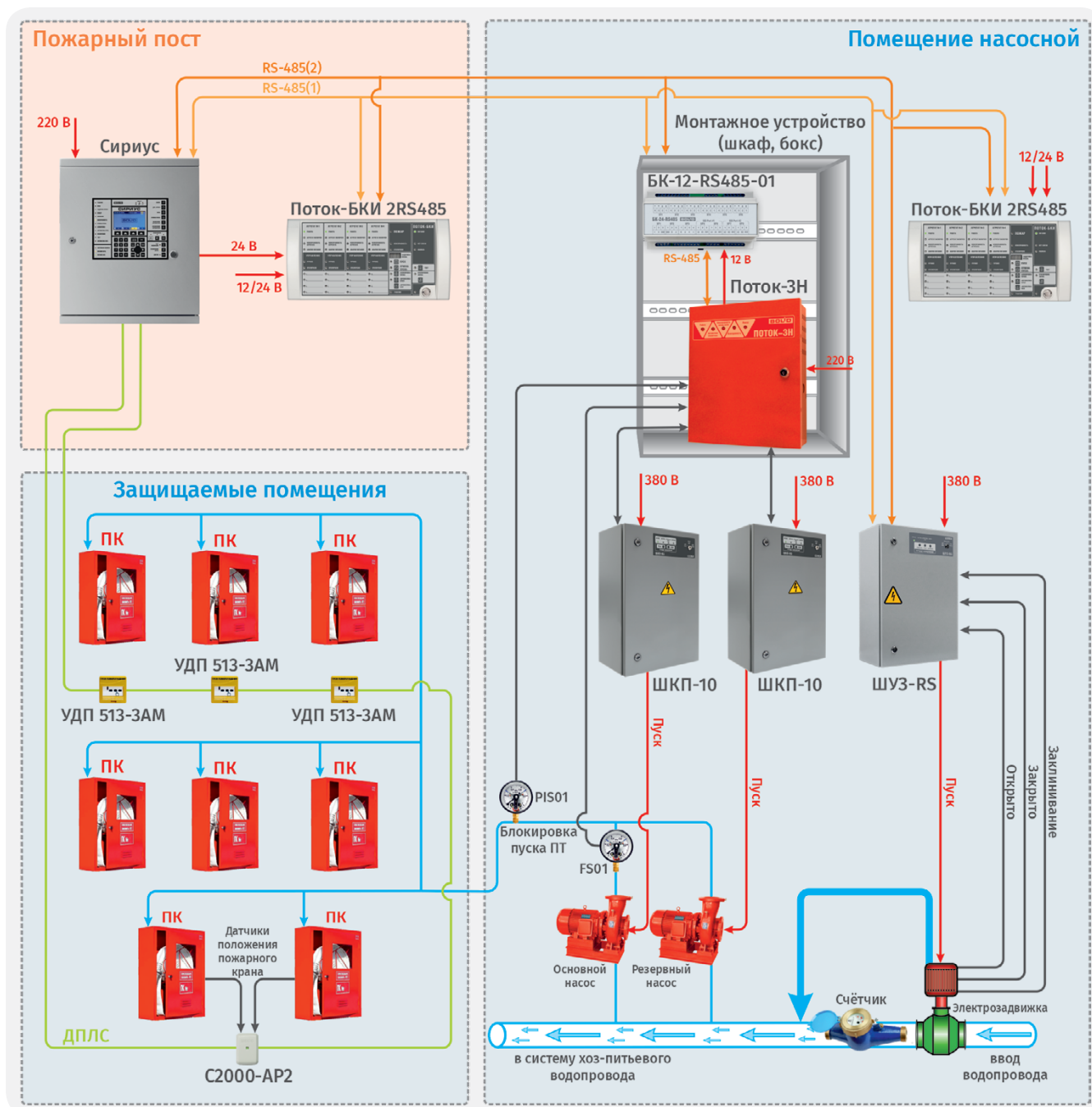
Рисунок 24. Внутренний противопожарный водопровод
