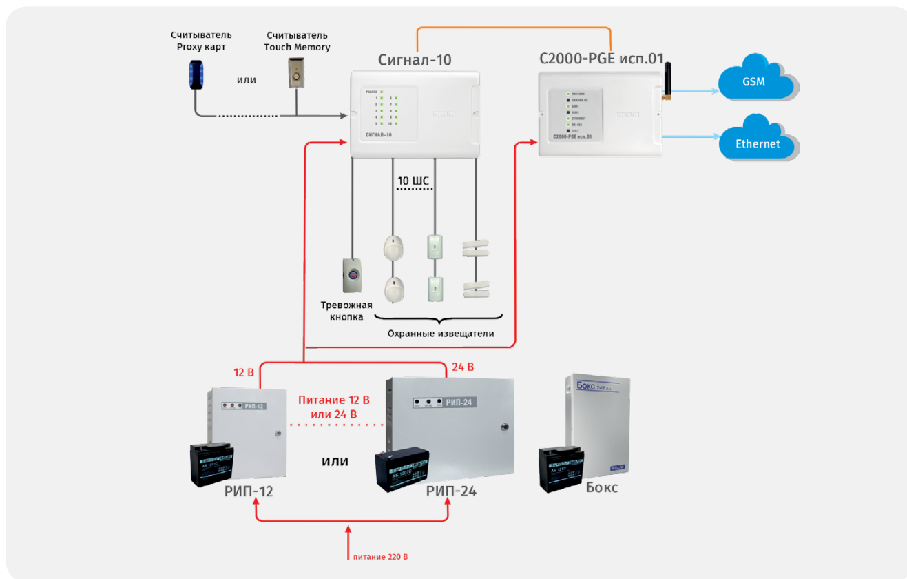
Рисунок 47. Система охранной сигнализации на базе прибора «Сигнал-10» и устройства «С2000-PGE исп.01»
