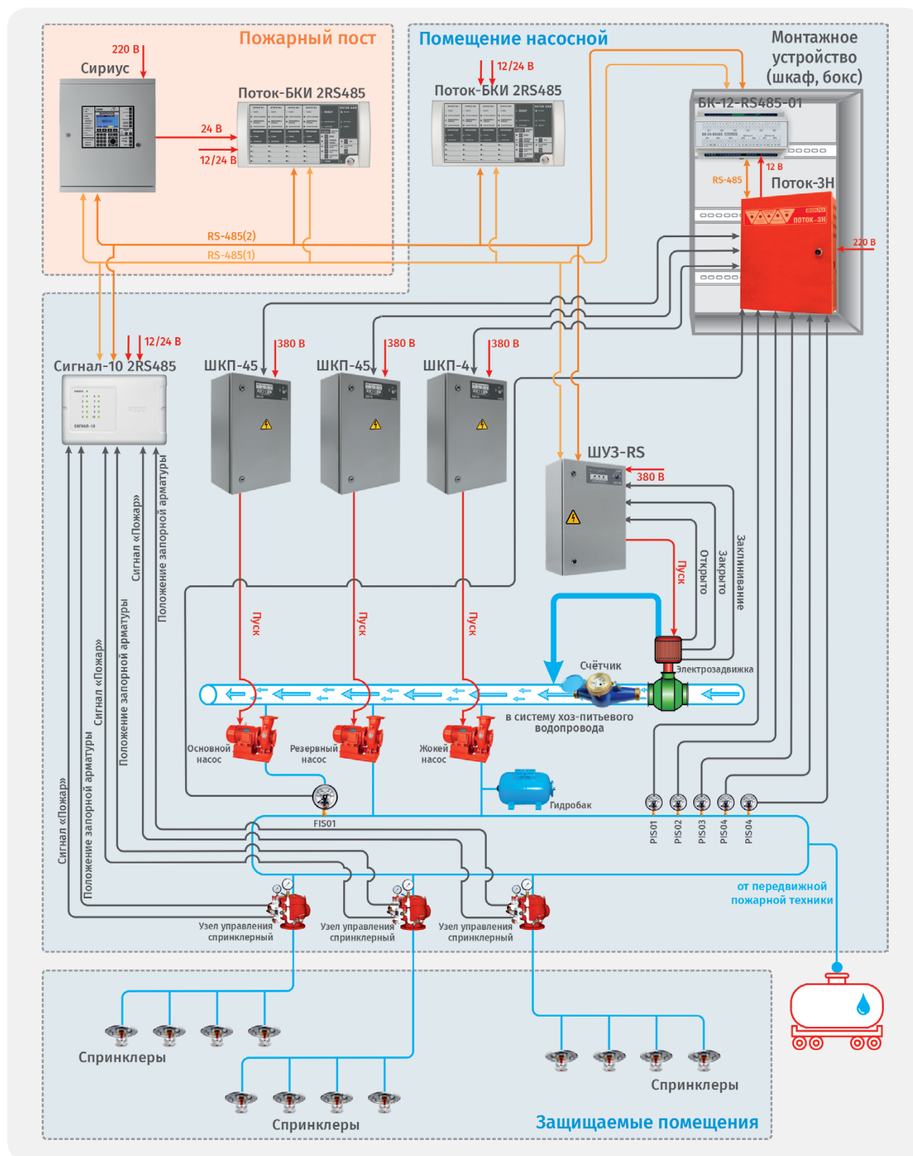
Рисунок 25. Автоматическая установка пожаротушения с тремя спринклерными секциями на направления (перед СПЖ).
