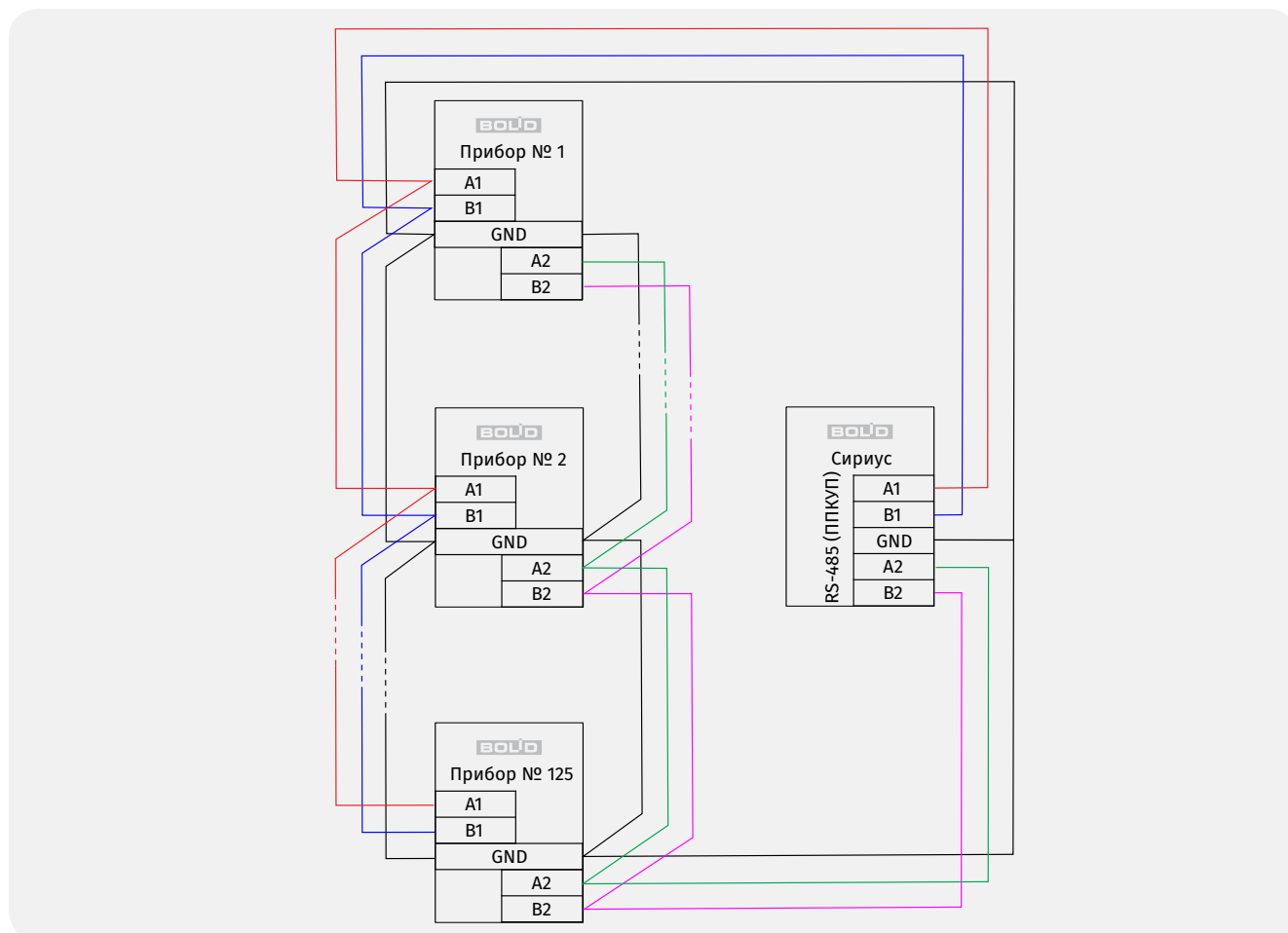
Рисунок 33. Структурная схема резервированного RS-485 интерфейса с топологией «кольцо»
