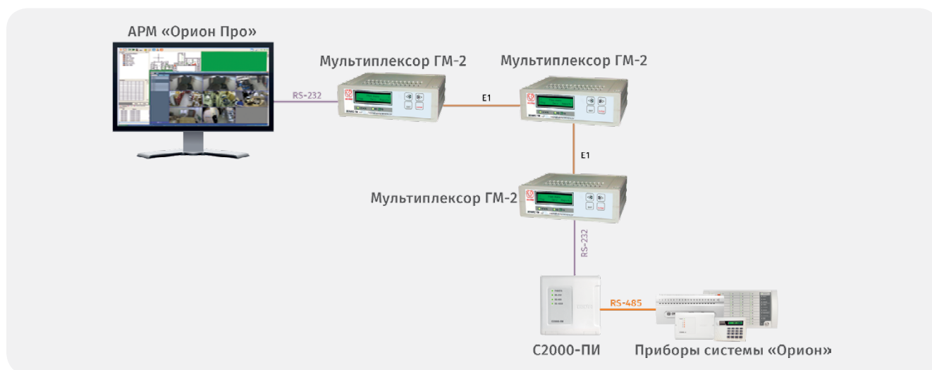
Рисунок 109. Структурная схема использования мультиплексора «ГМ-2» с АРМ «Орион Про» с подключением промежуточного мультиплексора (ремultipлексирование)
