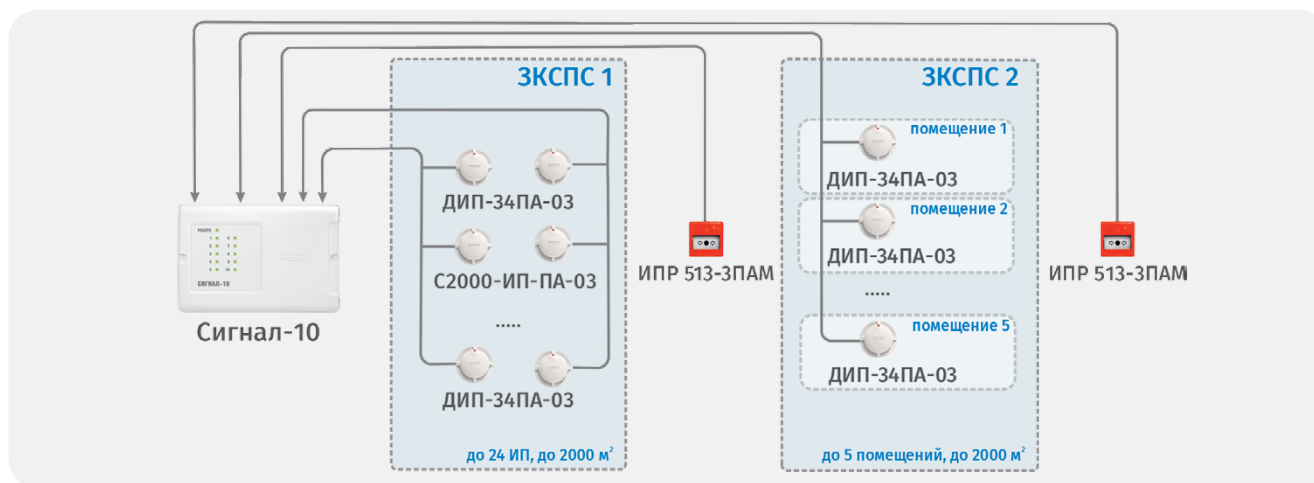
Рисунок 3. Организация линий и ЗКСПС в адресно-пороговых СПС
