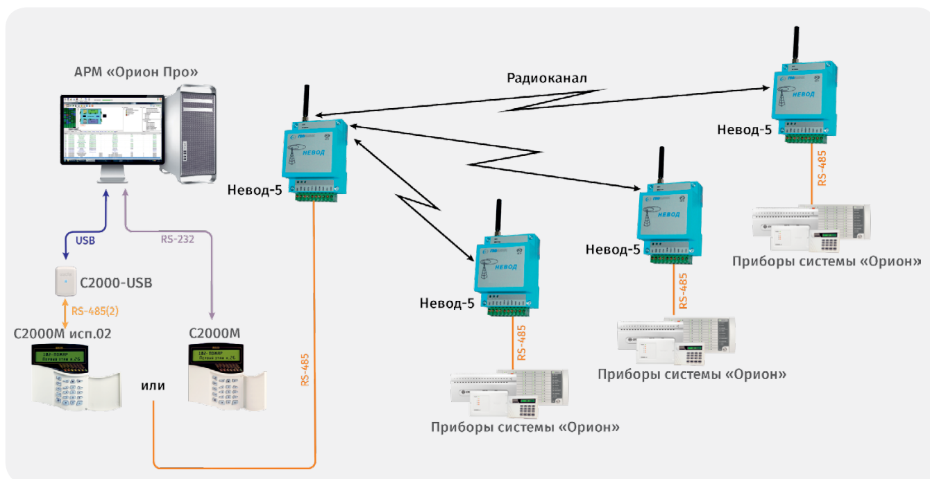
Рисунок 116. Структурная схема использования «Невод-5» с АРМ «Орион Про» и «С2000М»/ «С2000М исп.02», соединение «точка-многоточка»
