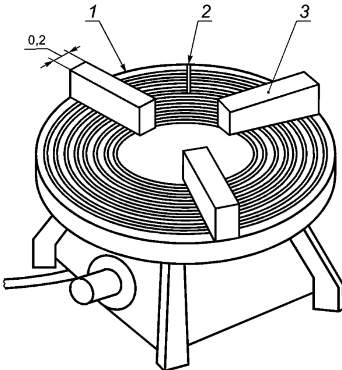
1 - плита; 2 - термопара; 3 - деревянные бруски
