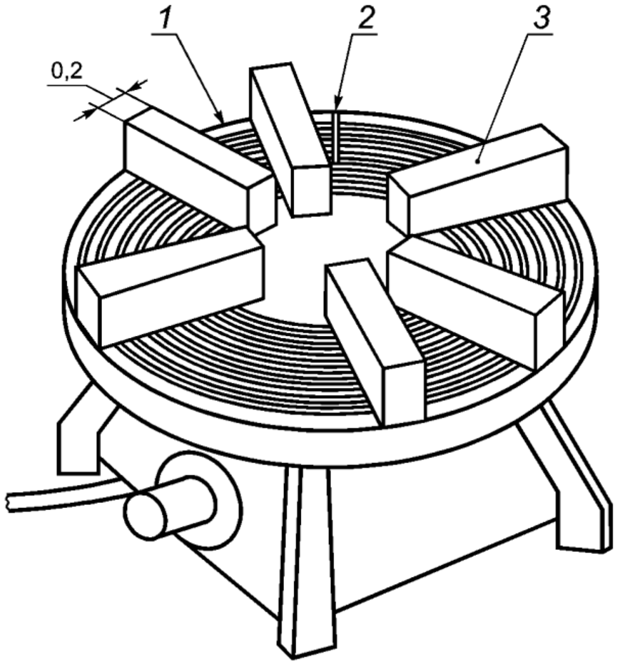
1 - плита; 2 - термопара; 3 - деревянные бруски
