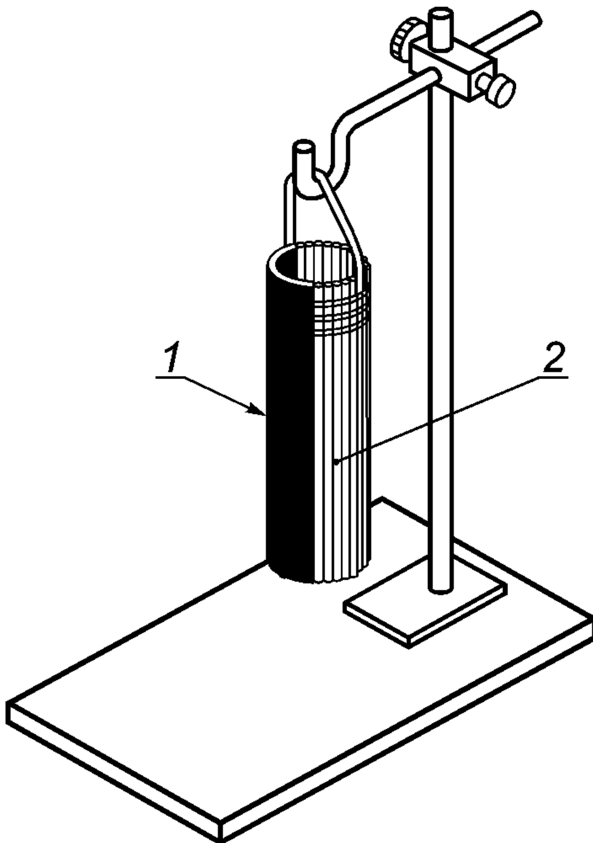
1 - изогнутый лист из негорючего материала; 2 - хлопковые фитили
