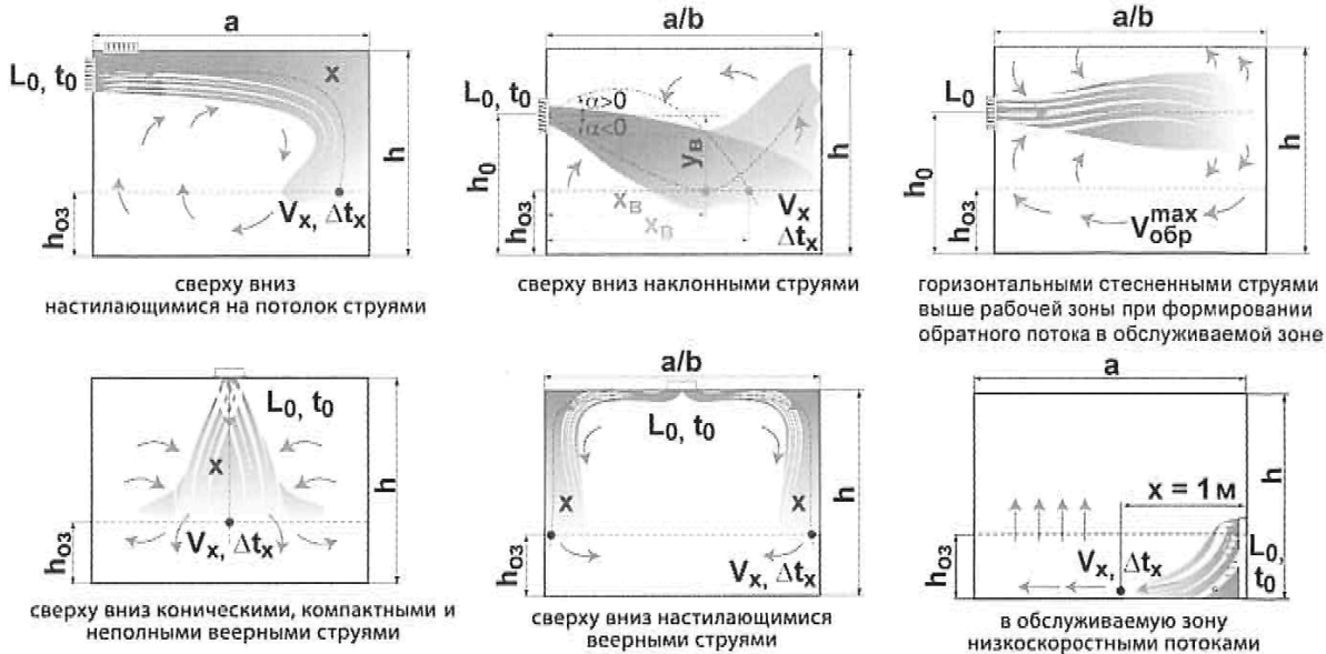
Рисунок Ж.1 – Основные схемы подачи приточного воздуха
