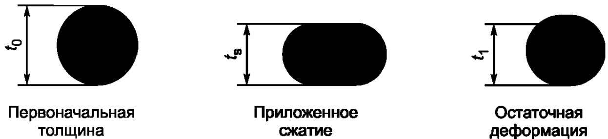
Рисунок 6 - Остаточная деформация при сжатии уплотнительного кольца
