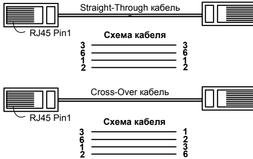
Рисунок 5 Типы Ethernet-кабелей
