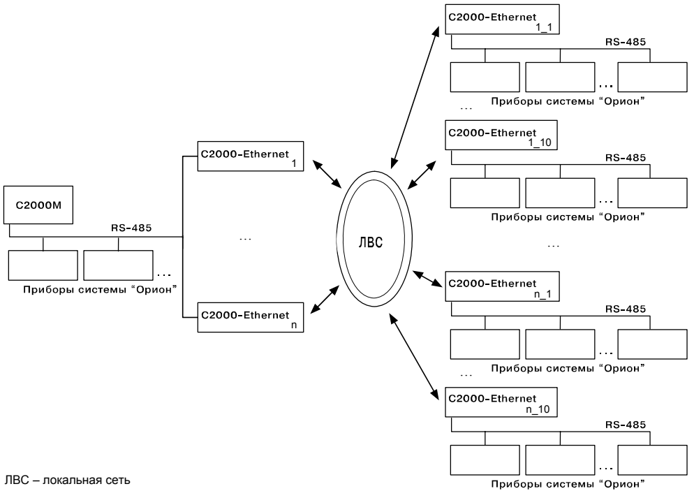
Рисунок 3 Типовая схема использования "C2000-Ethernet" с "C2000M"
