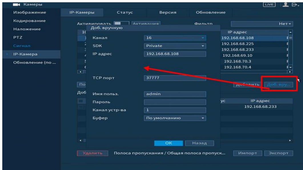
Рисунок 6.54 Настройка ручного добавления камер
