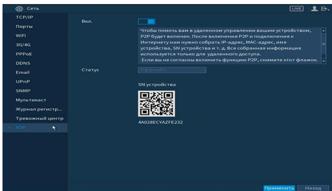
Рисунок 6.69 Интерфейс настройки «P2P»
