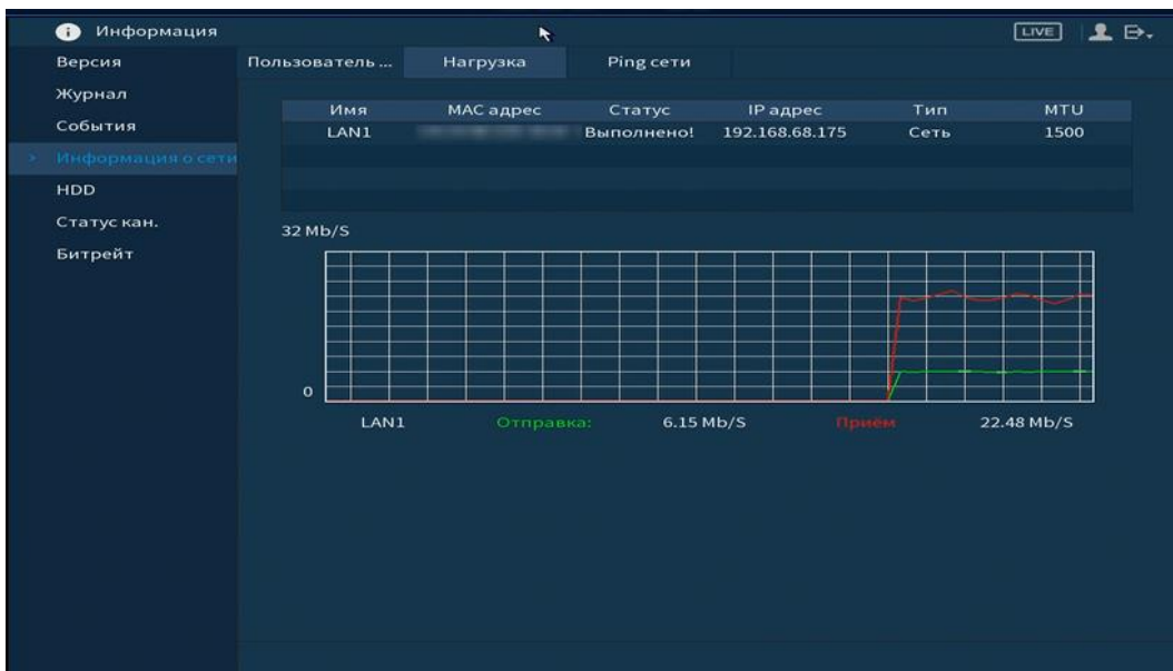
Рисунок 6.110 Интерфейс просмотра нагрузки
