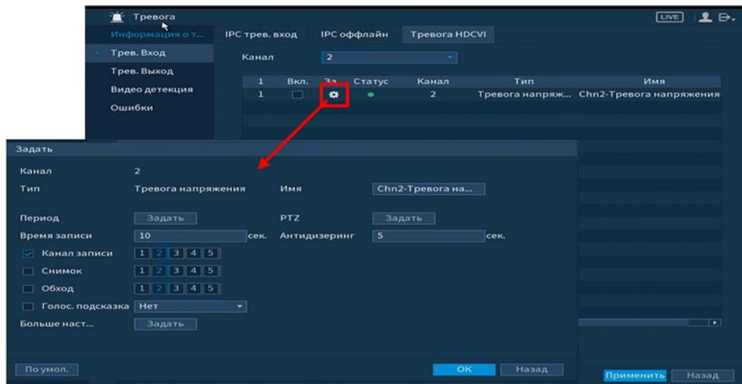
Рисунок 6.17 Настройка тревоги устройств HDCVI
