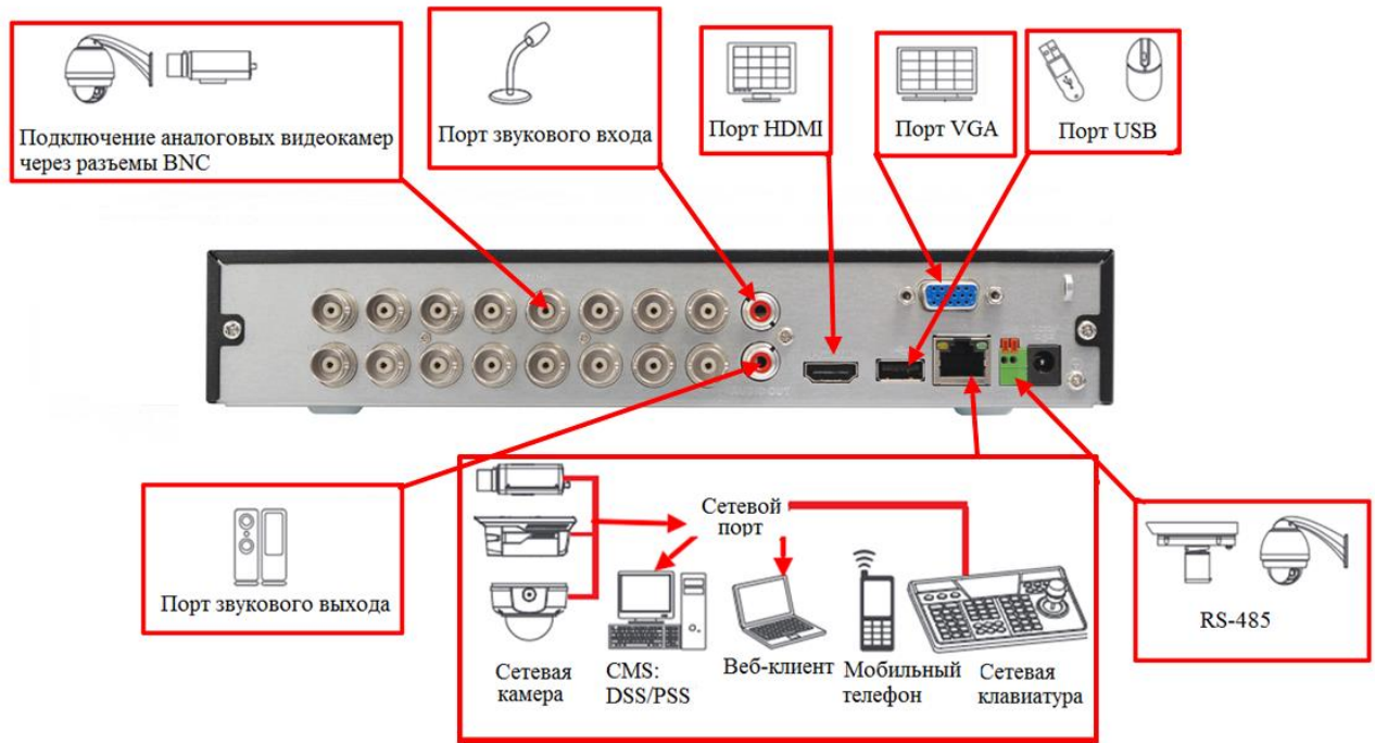
Рисунок 3.2 Внешний вид задней панели
