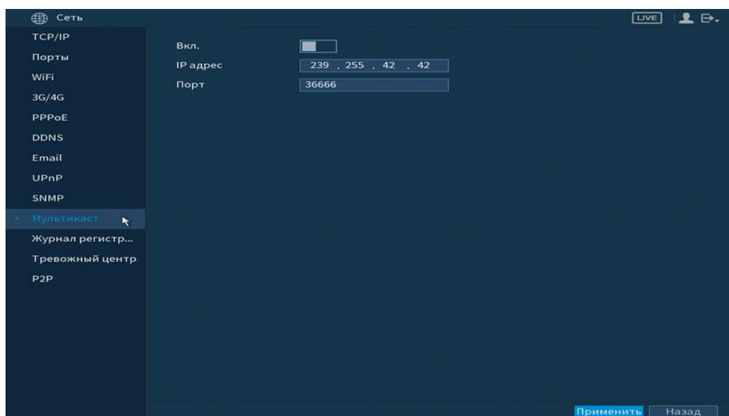
Рисунок 6.66 Интерфейс настройки «Мультикаст» Функции и диапазоны значений параметров (Таблица 6.17).
