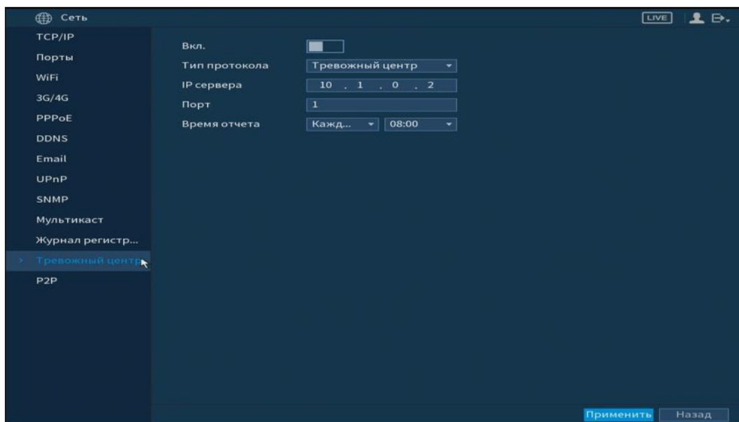
Рисунок 6.68 Интерфейс настройки «Трев. центр»
