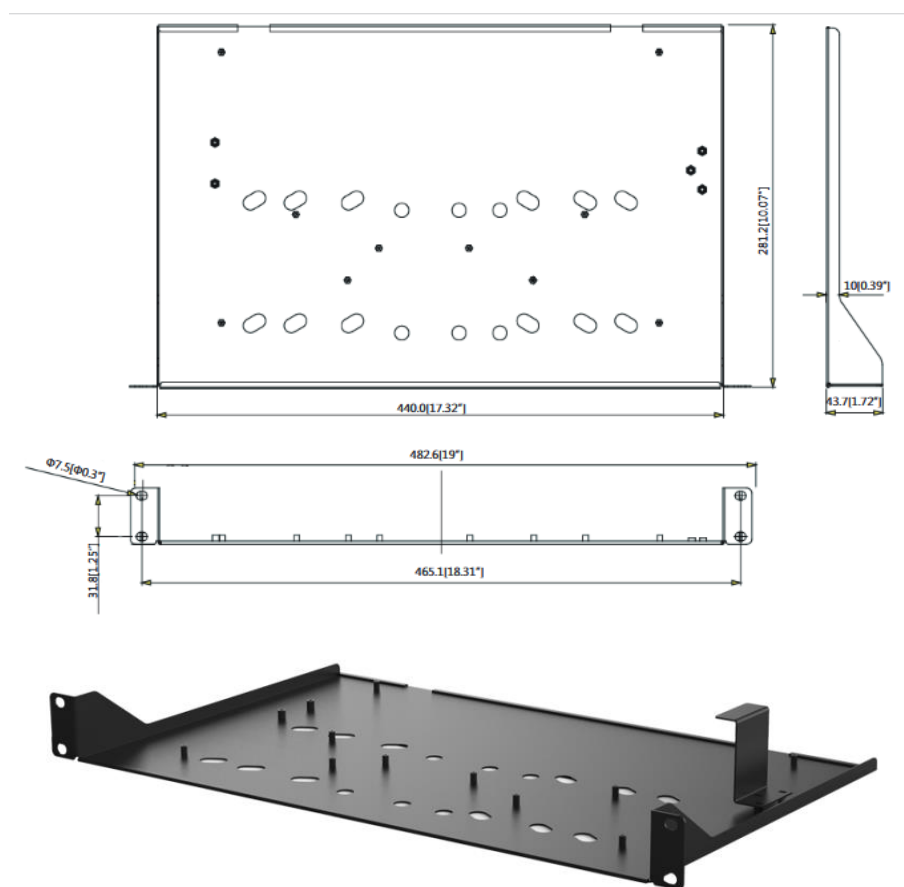
Рисунок 3.11 Внешний вид и габариты BR-111
