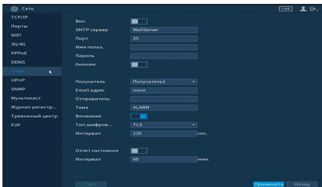
Рисунок 6.63 Интерфейс настройки «Email»
