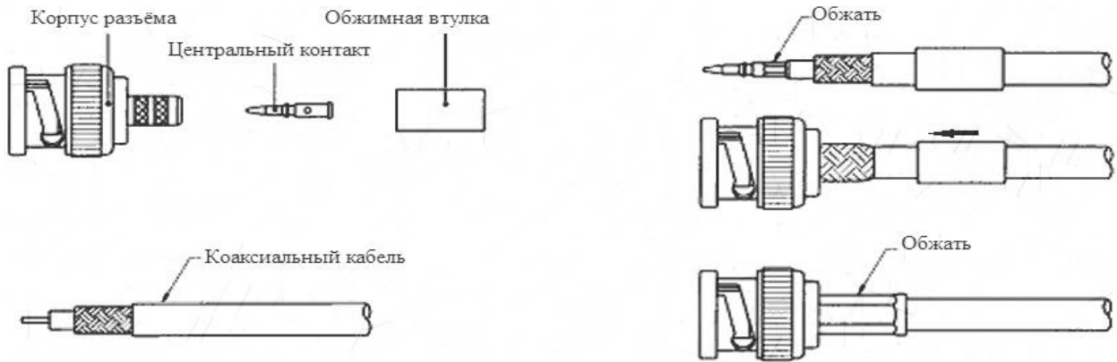
Рисунок 3.10 Схема обжима BNC
