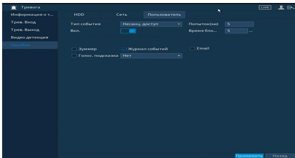
Рисунок 6.34 Интерфейс настройки тревожного выхода
