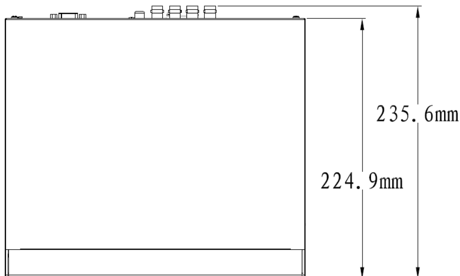
Рисунок 3.9 Габаритные размеры видеорегистратора
