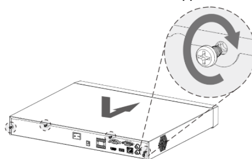
Рисунок 3.8 – Установка жесткого диска
