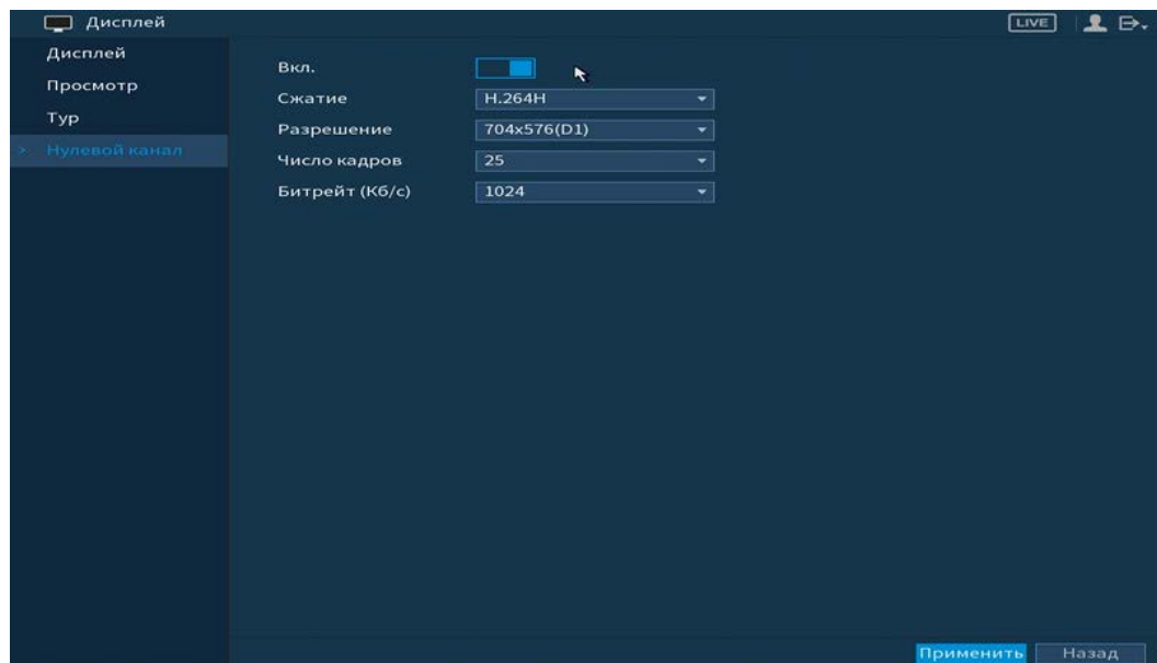
Рисунок 6.51 – Интерфейс настройки
