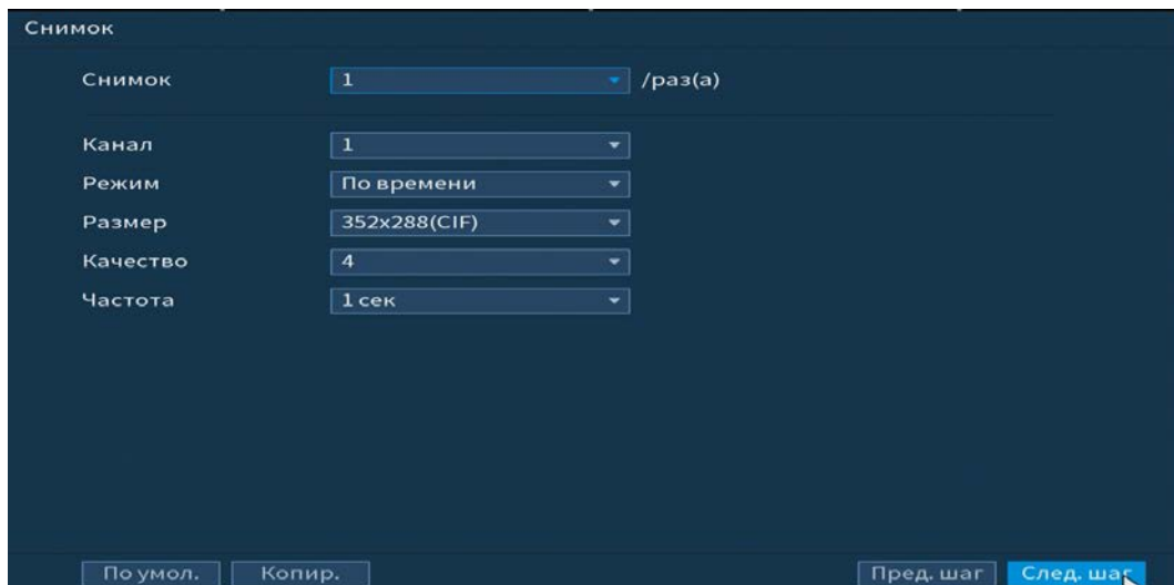
Рисунок 4.12 – Настройка снимка
