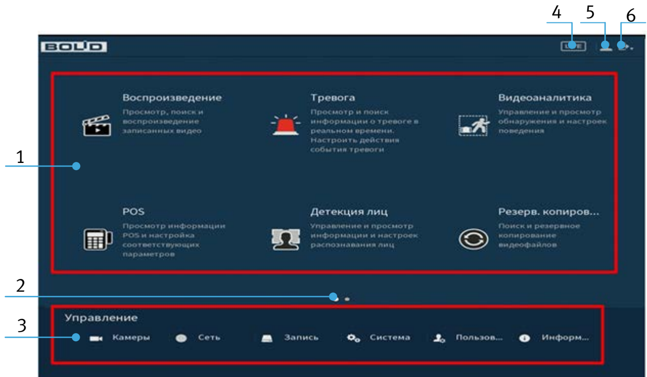
Рисунок 6.1 – Главное меню
