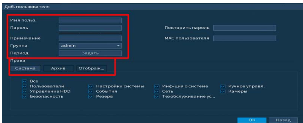
Рисунок 6.112 – Добавление пользователя
