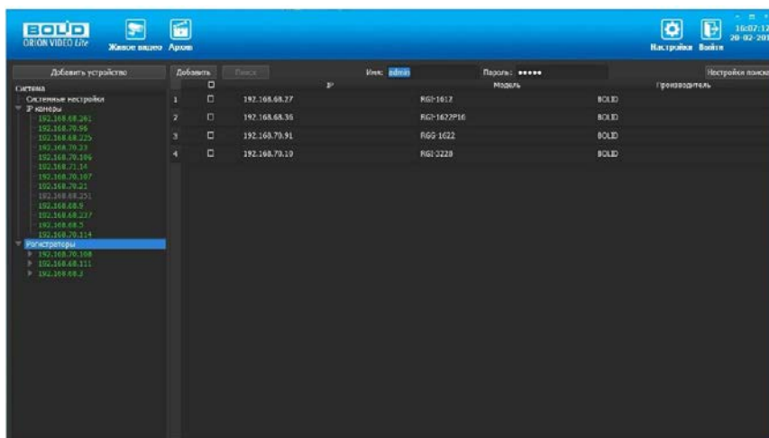
Рисунок 11.4 – Таблица результатов
