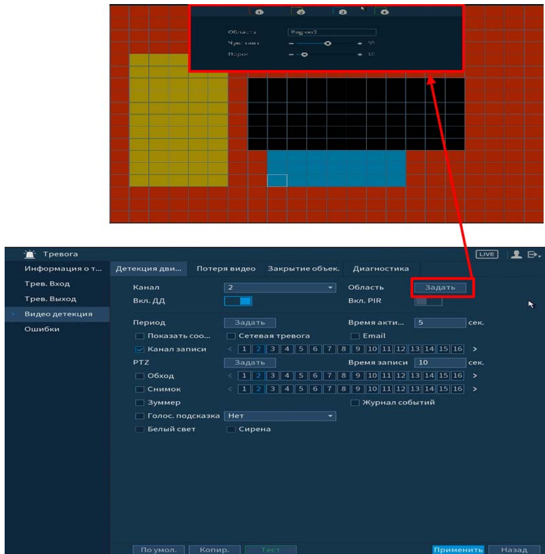
Рисунок 6.18 – Настройка области
