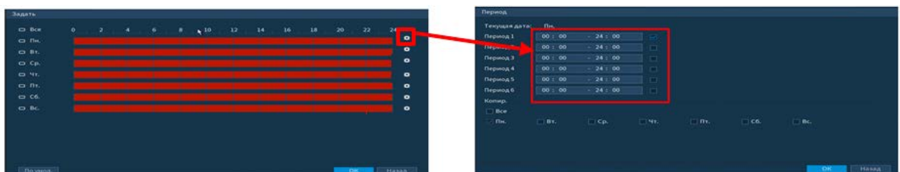
Рисунок 6.45 – Настройка расписания
