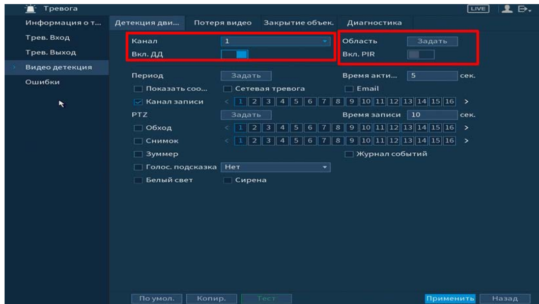
Рисунок 6.17 – Настройка события
