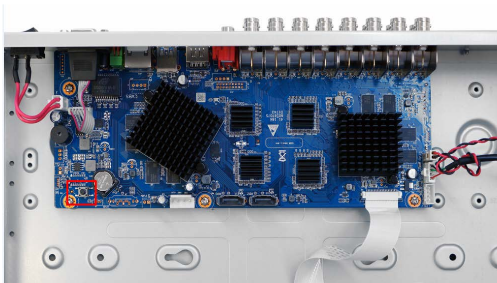
Рисунок 6.107 – Возможный пример нахождения кнопки сброса
