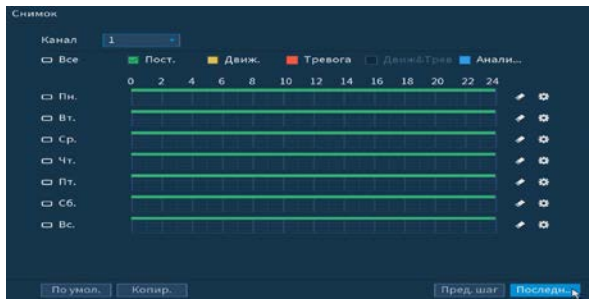
Рисунок 4.19 – Настройка расписания
