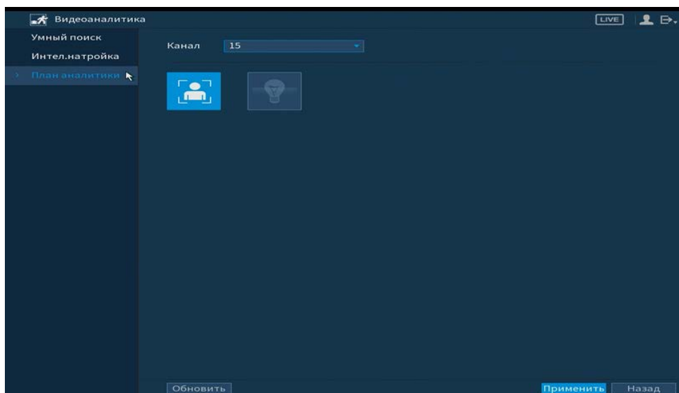
Рисунок 6.39 – Выбор функции
