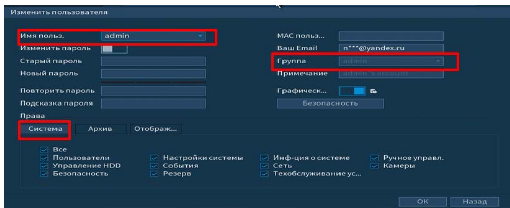
Рисунок 6.111 – Назначение прав
