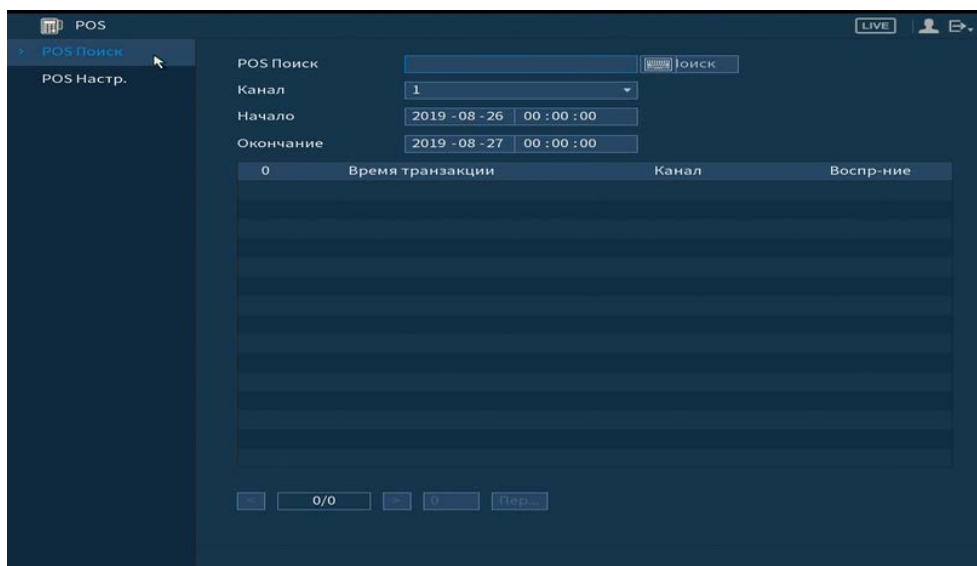
Рисунок 6.40 – Интерфейс поиска
