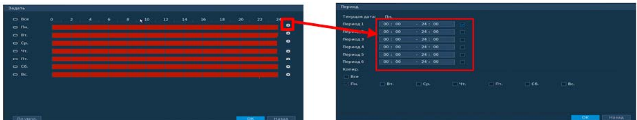
Рисунок 6.35 – Настройка расписания
