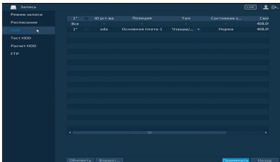
Рисунок 6.90 – Интерфейс настройки
