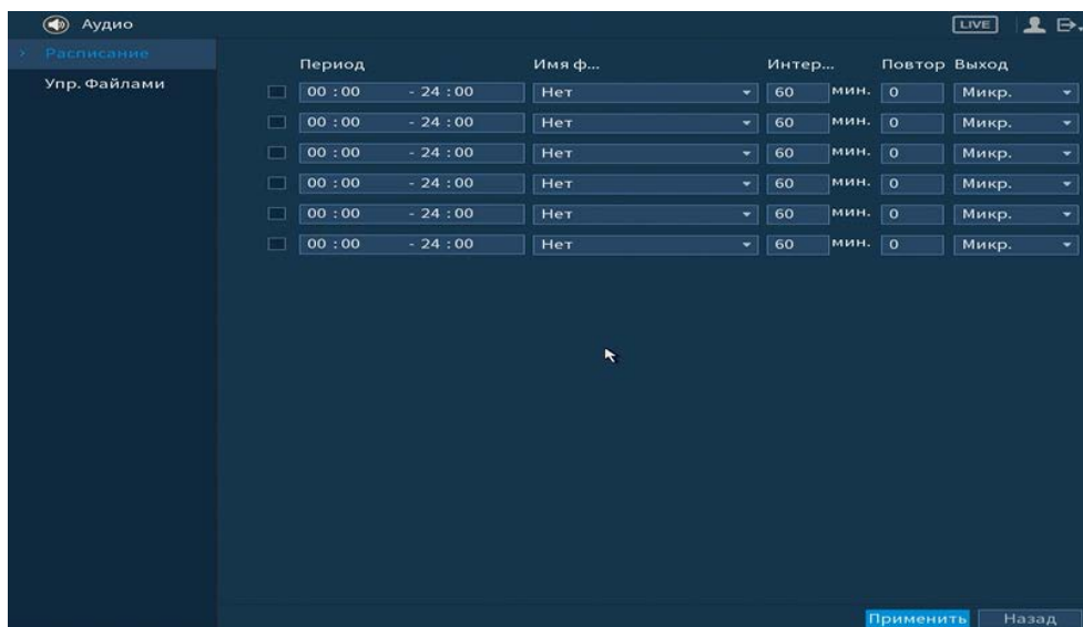
Рисунок 6.52 – Установка расписания
