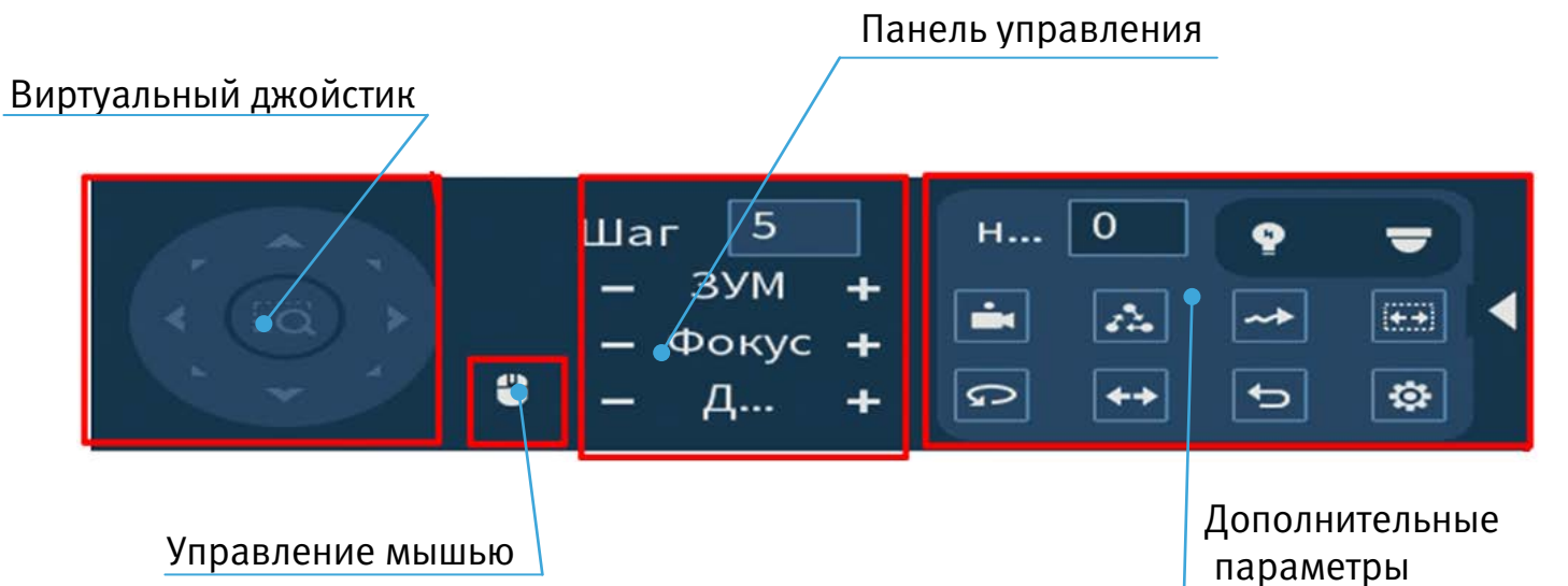
Рисунок 5.3 – Панель PTZ-управления
