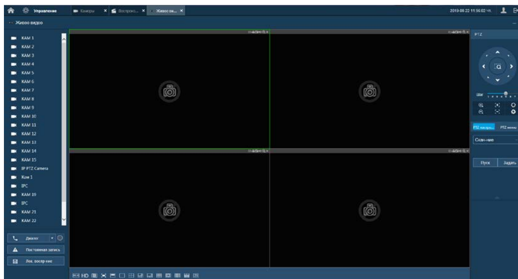
Рисунок 10.3 – Режим просмотра
