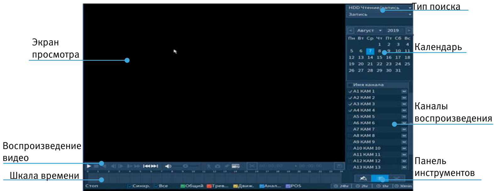
Рисунок 6.2 – Просмотр архива
