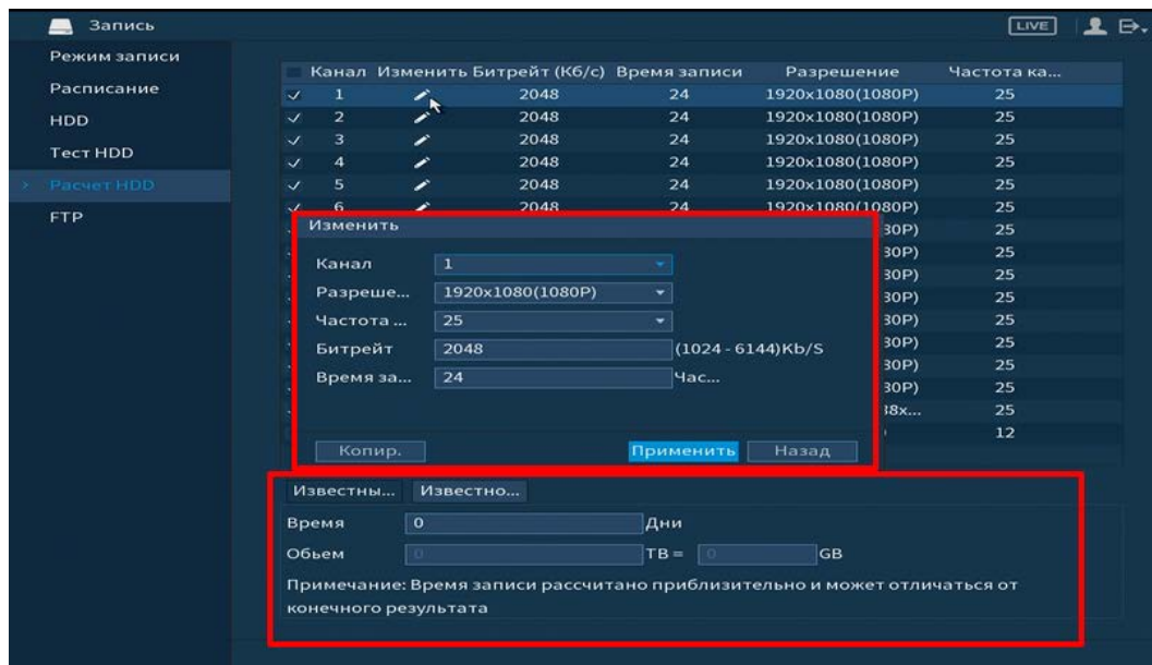
Рисунок 6.94 – Расчет объема
