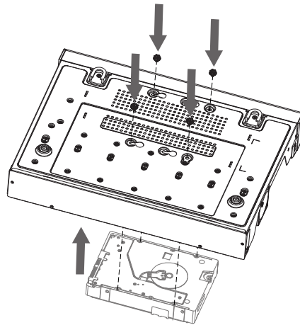
Рисунок 4.4 – Установка жесткого диска
