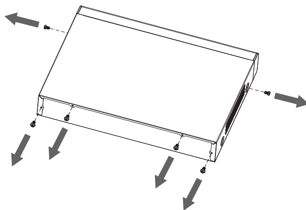
Рисунок 4.2 – Установка жесткого диска
