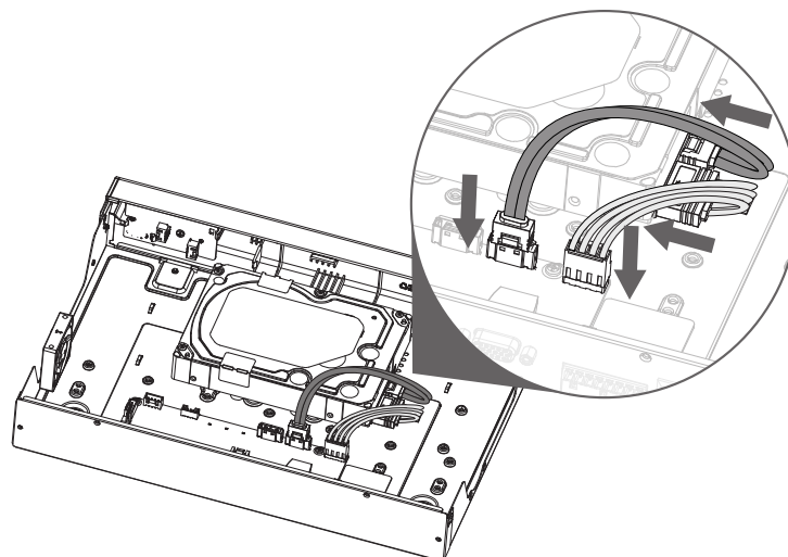
Рисунок 4.5 – Установка жесткого диска
