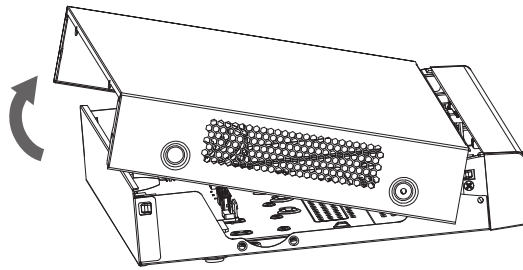
Рисунок 4.3 – Установка жесткого диска
