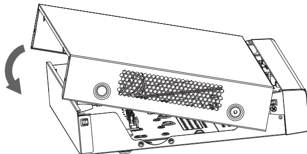
Рисунок 4.6 – Установка жесткого диска
