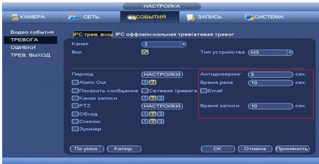
Рисунок 8.82 Установка настроек.
