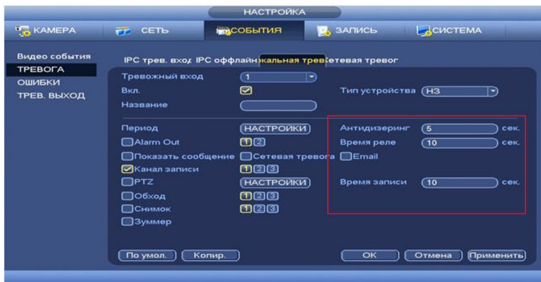
Рисунок 8.92 Установка настроек.
