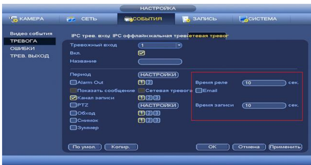
Рисунок 8.98 Установка настроек.
