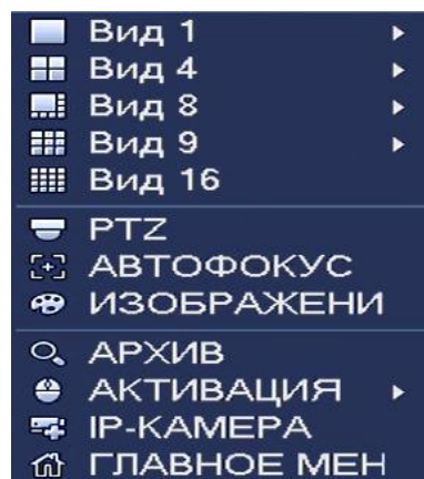
Рисунок 7.1 Контекстное меню.
