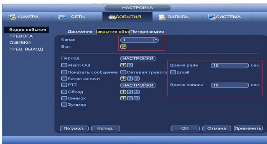
Рисунок 8.76 Установка настроек.
