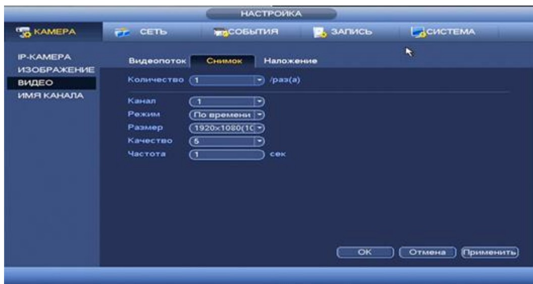
Рисунок 8.40 Настройка снимка.
