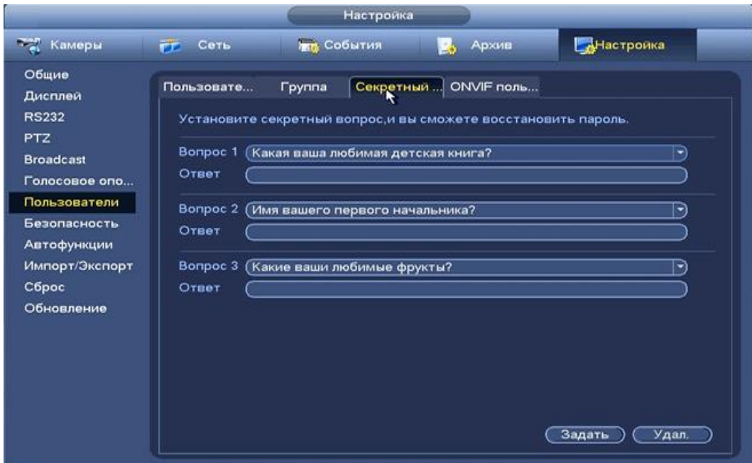
Рисунок 8.134 Интерфейс настройки
