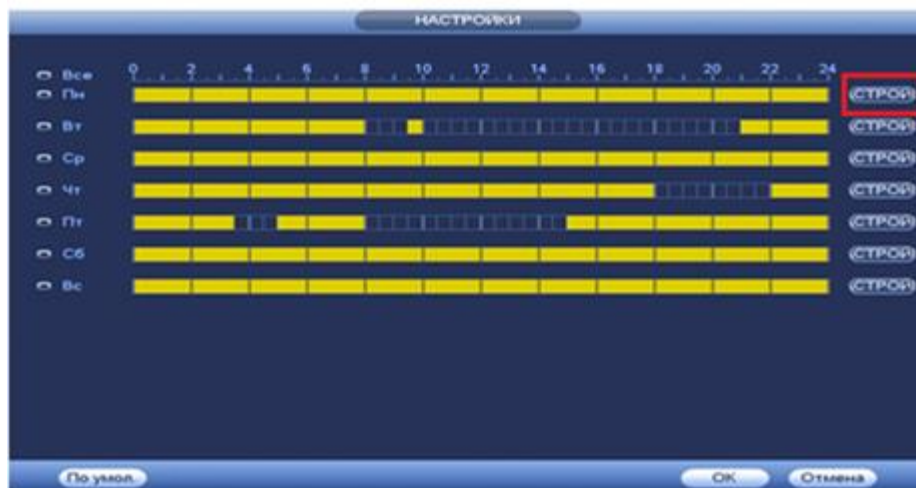
Рисунок 8.61 Настройка расписания.
