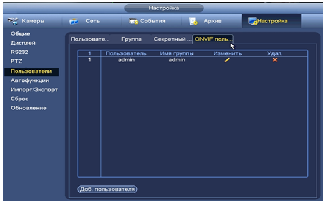
Рисунок 8.135 Настройка ONVIF.
