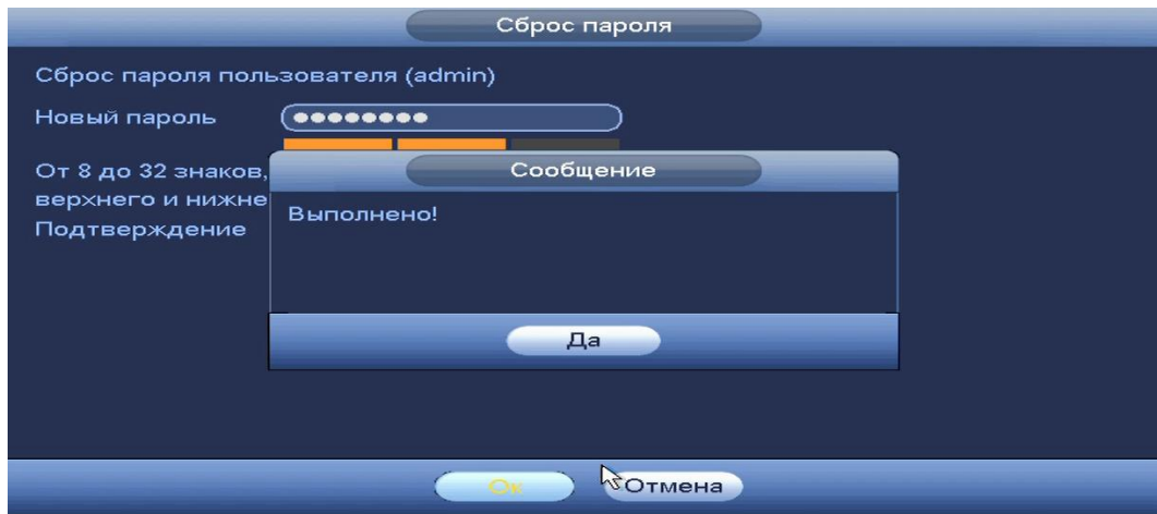
Рисунок 8.148 Ввод пароля.
