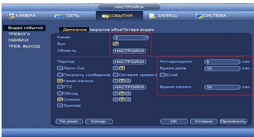
Рисунок 8.64 Установка настроек
