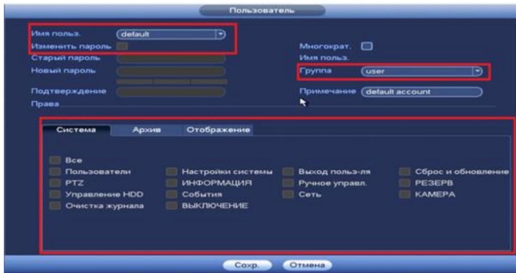
Рисунок 8.130 Назначение прав.
