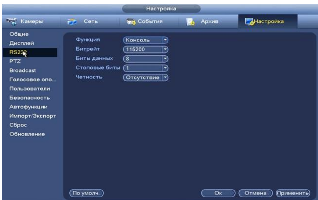
Рисунок 8.126 Интерфейс настройки
