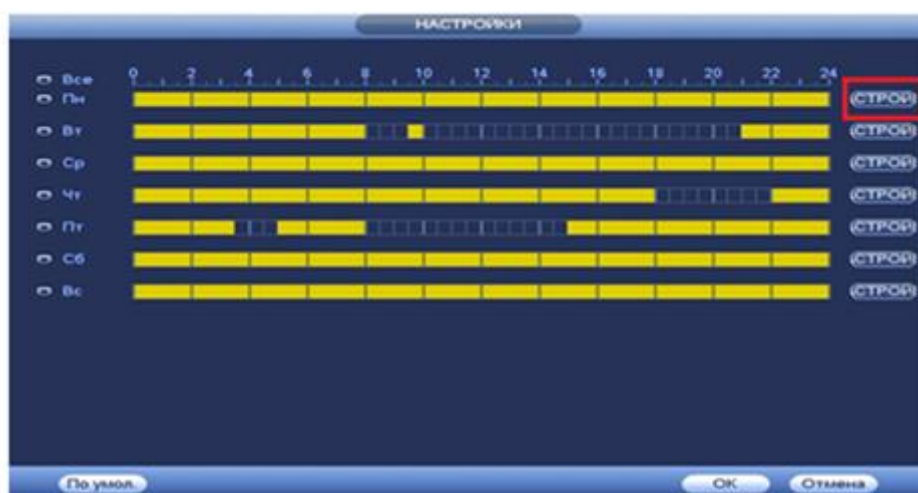
Рисунок 8.79 Настройка расписания.
