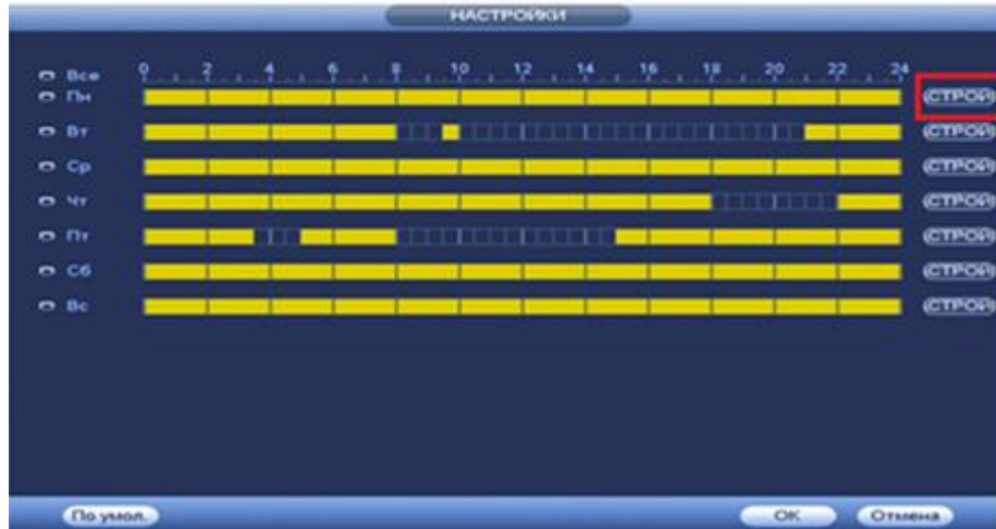
Рисунок 8.67 Настройка расписания.
