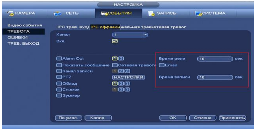
Рисунок 8.86 Установка настроек
