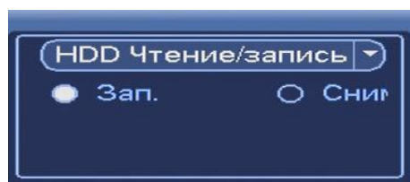
Рисунок 7.17 Тип поиска.
