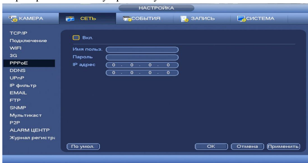
Рисунок 8.48 Интерфейс настройки «PPPoE».
