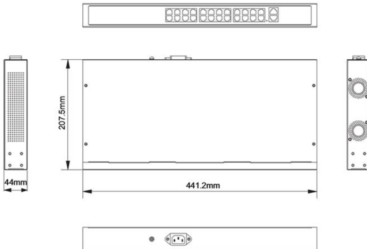
Рисунок 2 – Габаритные размеры
