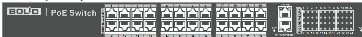
Рисунок 1 – Передняя панель
