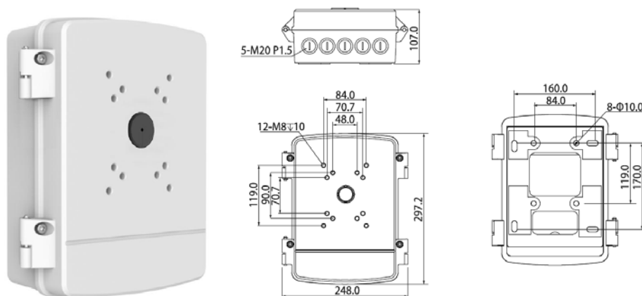
Рисунок 5.5 — Монтажная коробка BR-203
