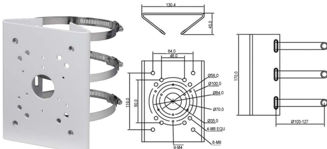
Рисунок 5.14 — Столбовой кронштейн BR-103
