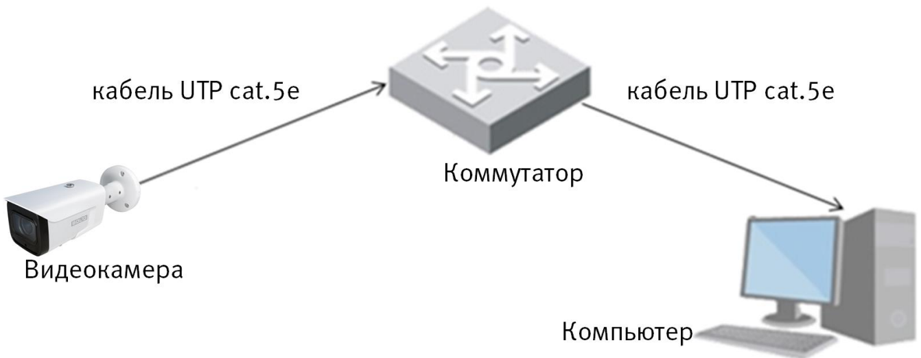
Рисунок 6.3 - Схема подключения видеокамеры к компьютеру через коммутатор
