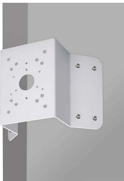
Рисунок 5.8 – Определение точек крепления кронштейна на установочной поверхности
