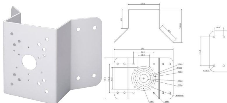
Рисунок 5.10 – Угловой кронштейн BR-102
