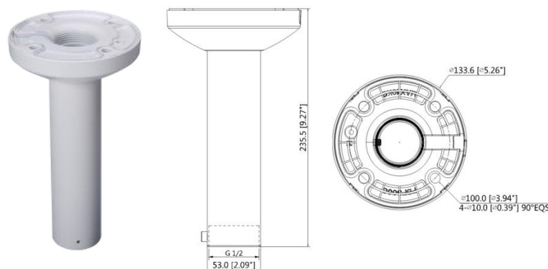
Рисунок 5.3 – Потолочный кронштейн BR-104
