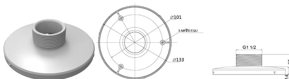
Рисунок 5.8 – Монтажный адаптер BR-304
