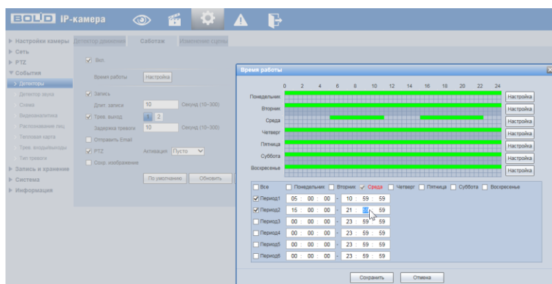
Рисунок 7.99 – Вкладка «Саботаж»: Время работы
