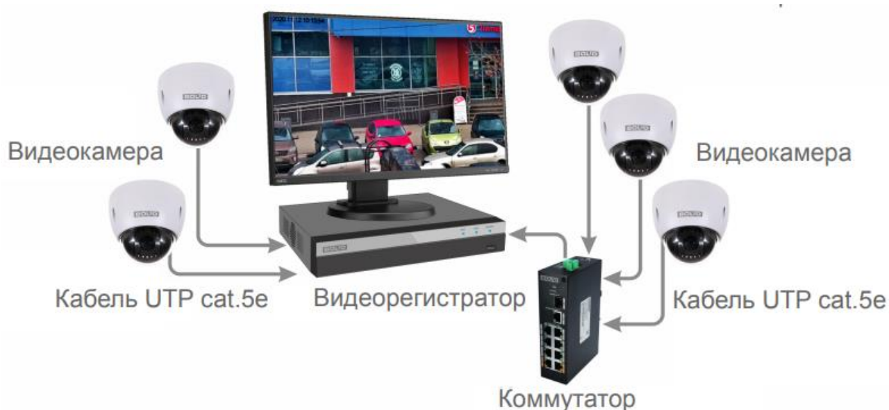
Рисунок 6.4 – Схема подключения видеокамеры к видеорегистратору
