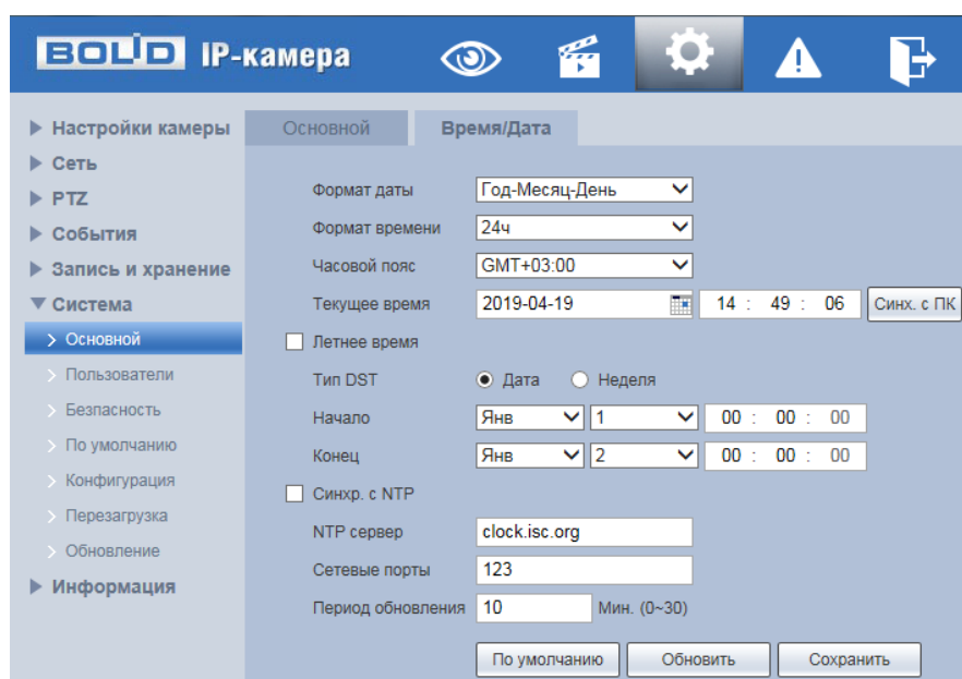
Рисунок 7.147 – Вкладка «Дата/Время»
