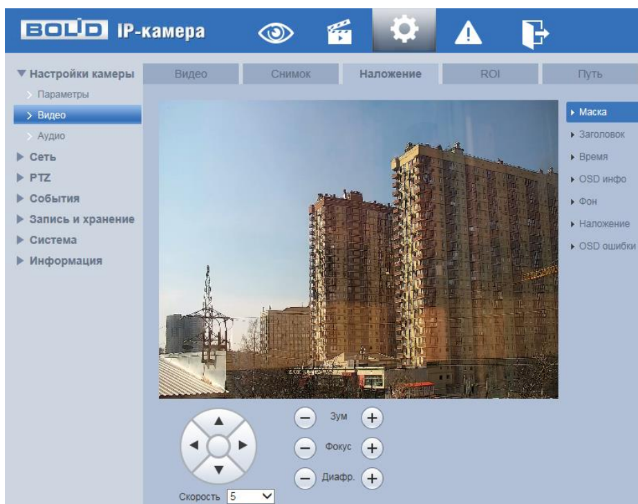
Рисунок 7.40 – Вкладка «Наложение»
