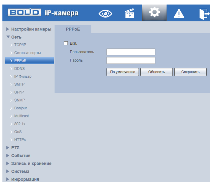
Рисунок 7.56 – Подпункт меню «PPPoE»
