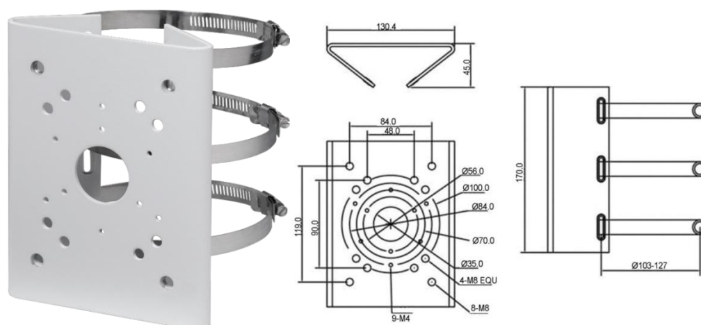
Рисунок 5.15 – Столбвой кронштейн BR-103
