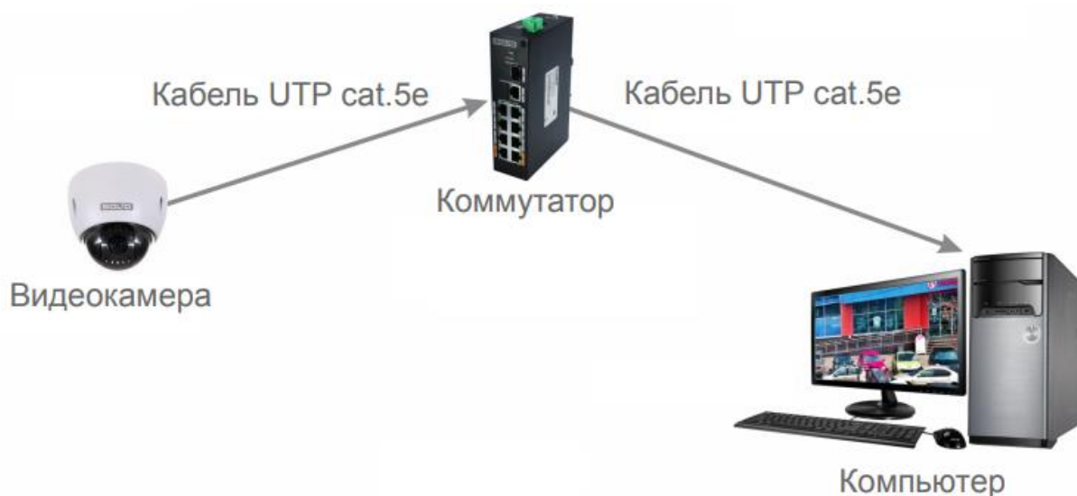
Рисунок 6.3 – Схема подключения видеокамеры к компьютеру через коммутатор
