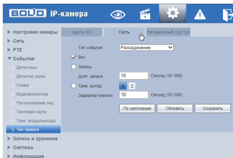
Рисунок 7.127 – Вкладка «Сеть»
