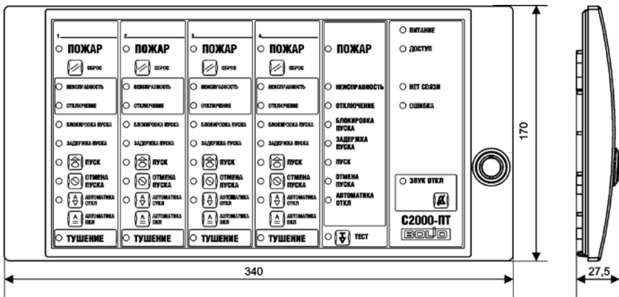
Вид сзади
