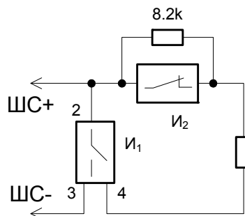
Схема подключения дымовых и тепловых извещателей, тип шлейфа 2
