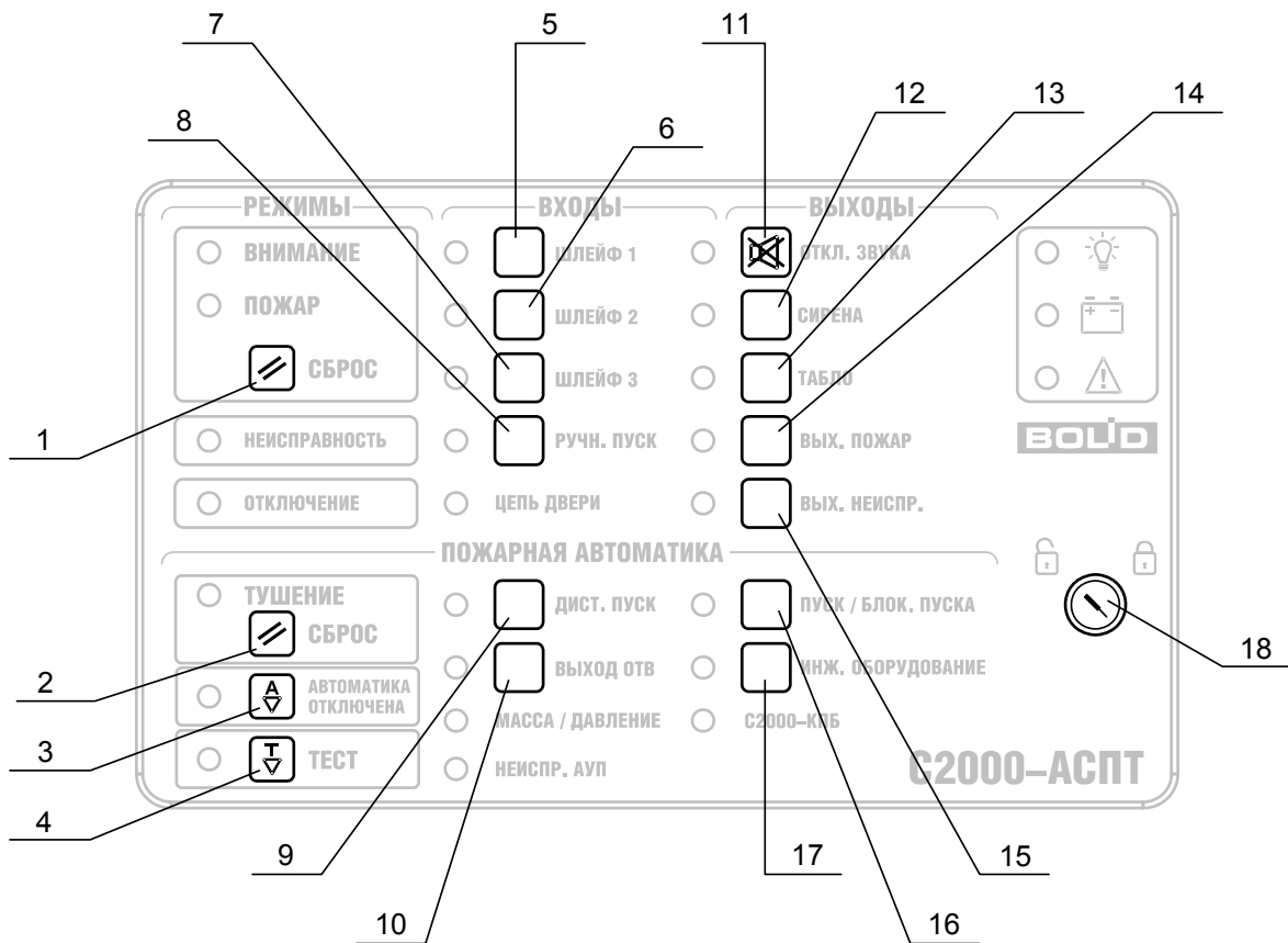
Рисунок 2.2 Расположение кнопок
