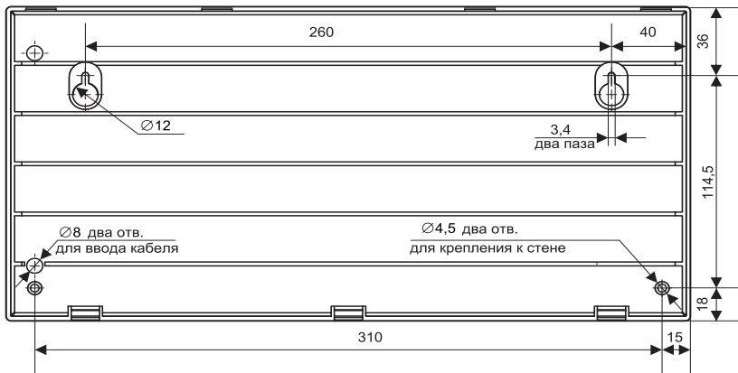
Рисунок 1. Внешний вид, габаритные и установочные размеры блока «С2000-ПТ»
