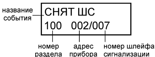
Рисунок 3.3 Пример экрана пульта при нажатии клавиши «1»
