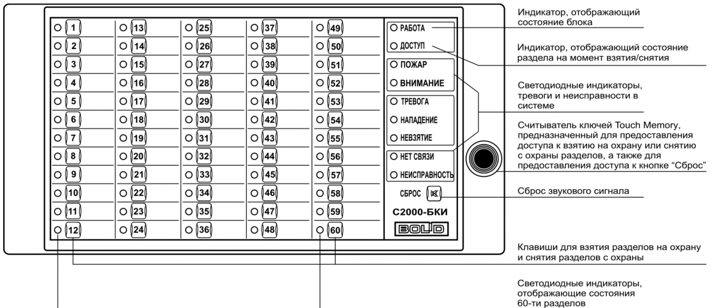
Рисунок 3.13 Внешний вид, органы индикации и управления блока С2000-БИ исп.02
