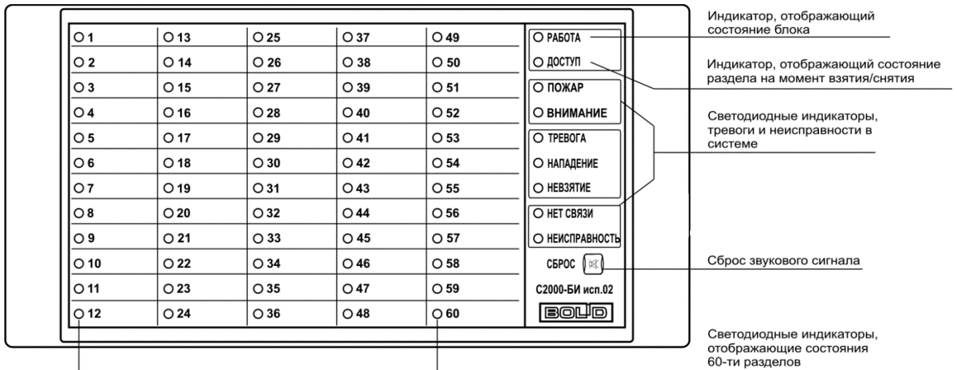
Рисунок 3.12 Внешний вид, органы индикации и управления блока С2000-БИ исп.02
