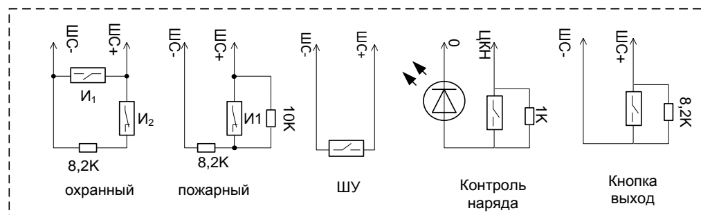
Рисунок 6. Подключение ШС, ШУ
